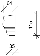
Karniis Šabloon võtta originaalilt M1:5
