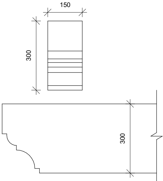
Päriniots Šabloon võtta originaalilt M1:5
