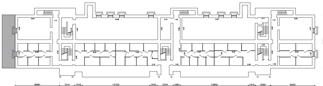
KELDRIKORRUSE PLAAN
