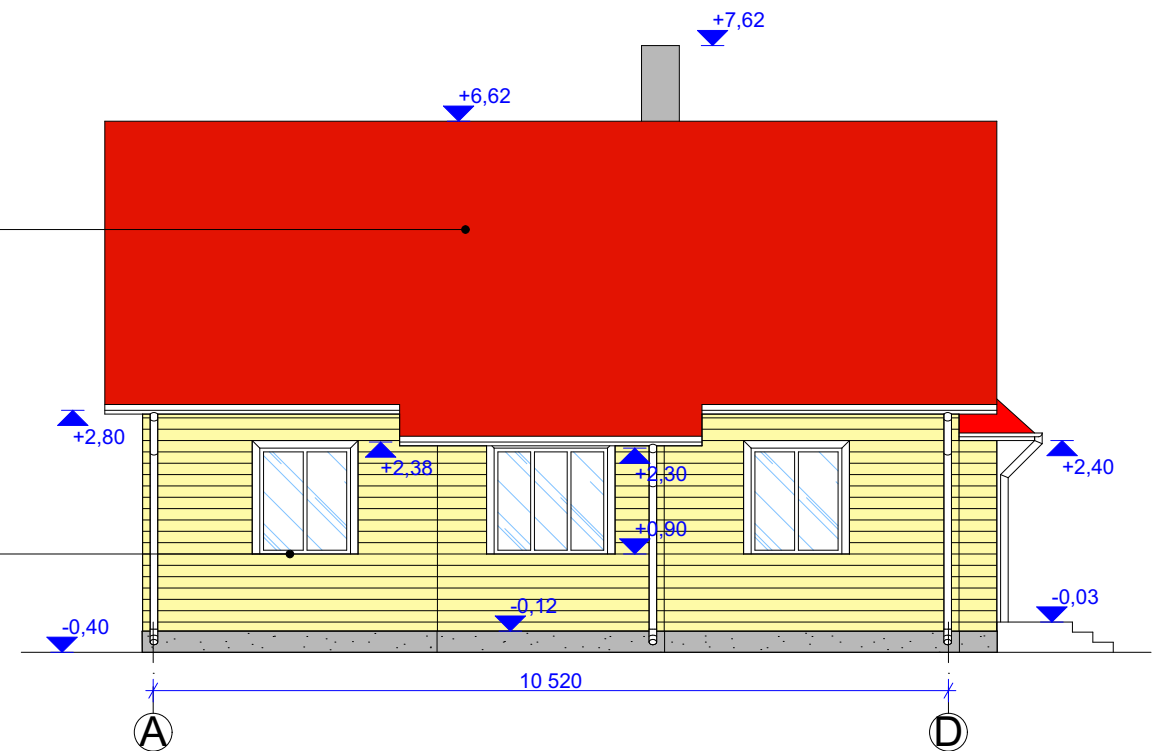
VAADE 2-2
