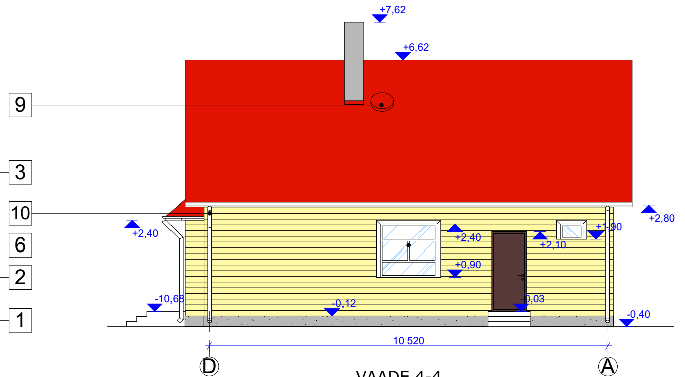
VAADE 4-4
