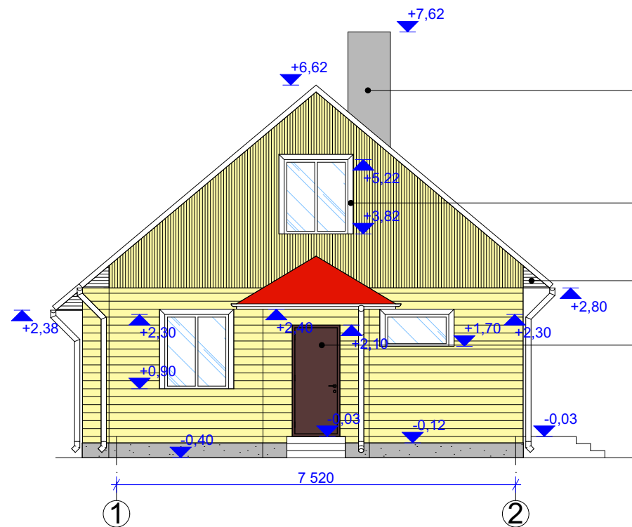
VAADE 1-1
