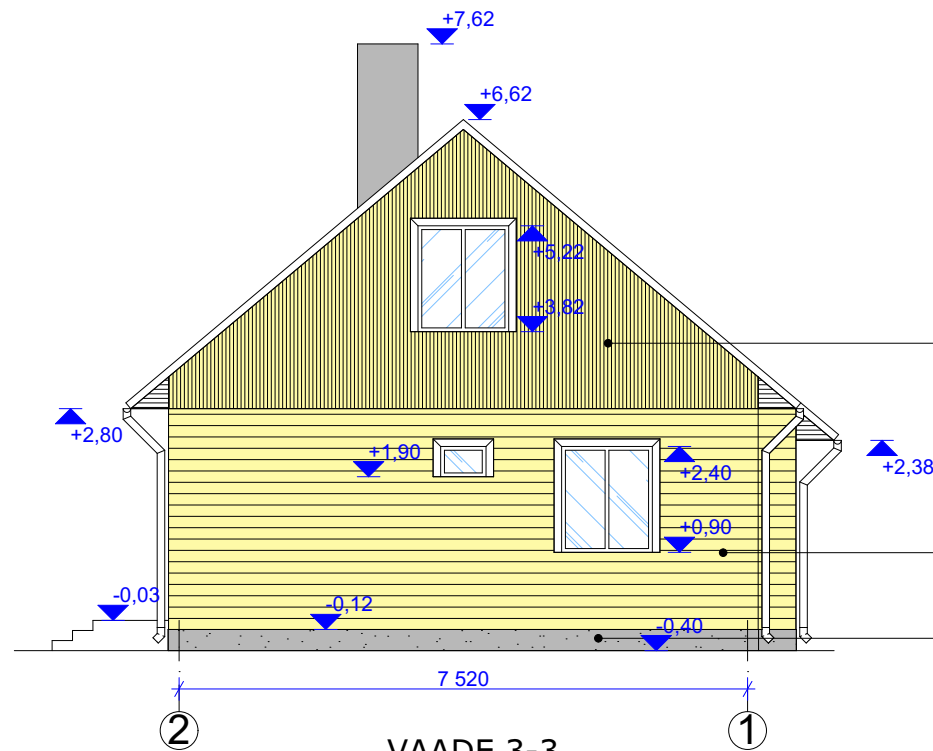
VAADE 3-3
