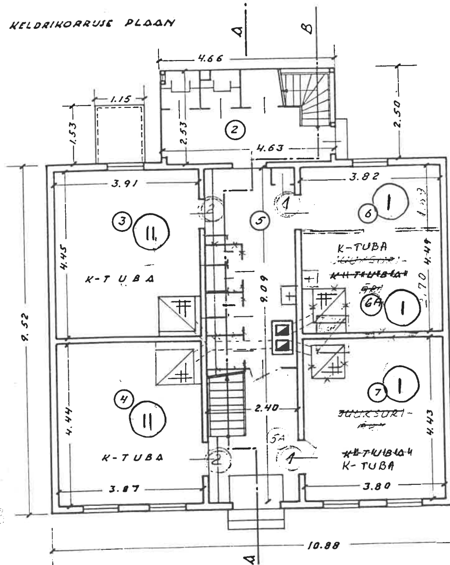
ESIMESE KORRUSE PLaan
