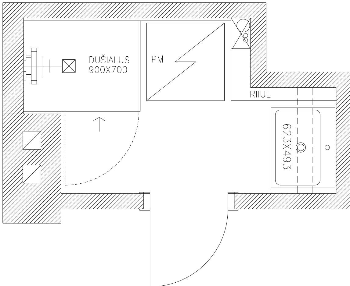
VANNITOA PLAANID DUŠIALUSEGA 08.03.2026
