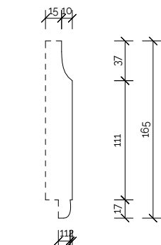
Rõhtlaudise profiil
