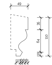
Vahekarniisi profiil
