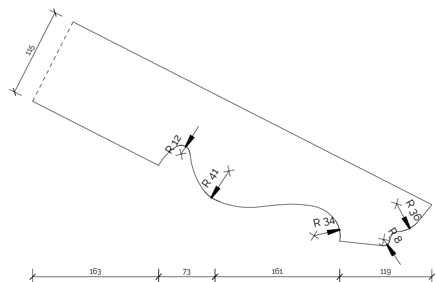
Põhimahu profileeritud sarikaots
