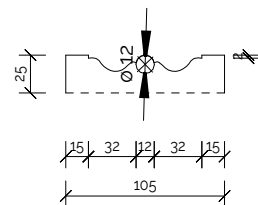
Akna piirdeliistu profiil
