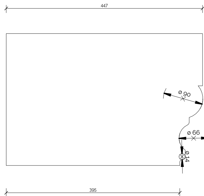
Profileeritud pärilin
