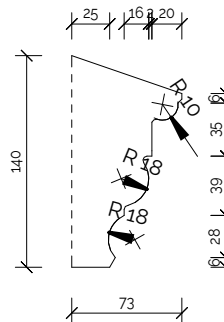
Aknapealne karniis
