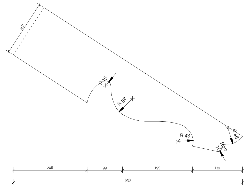
Põhimahu profileeritud sarikaots
