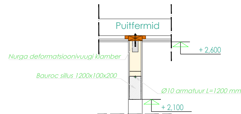
Vertikaalne lõige sillused
