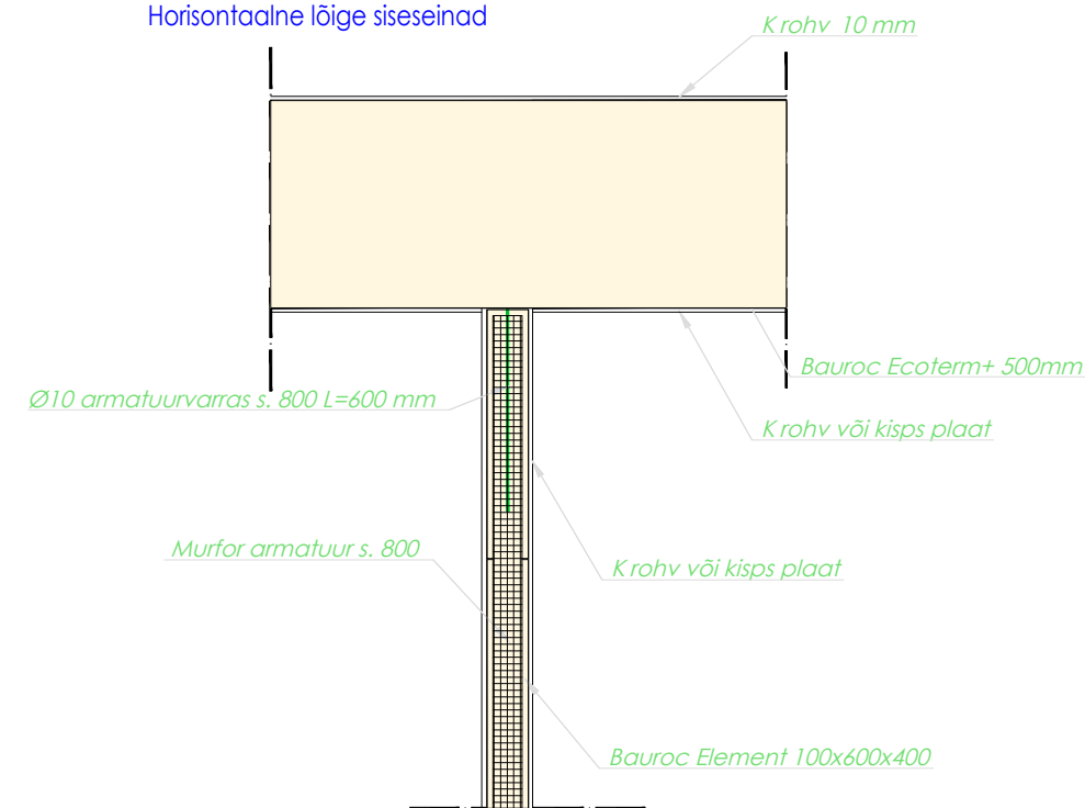
Horizontaalne lõige siseseinad
