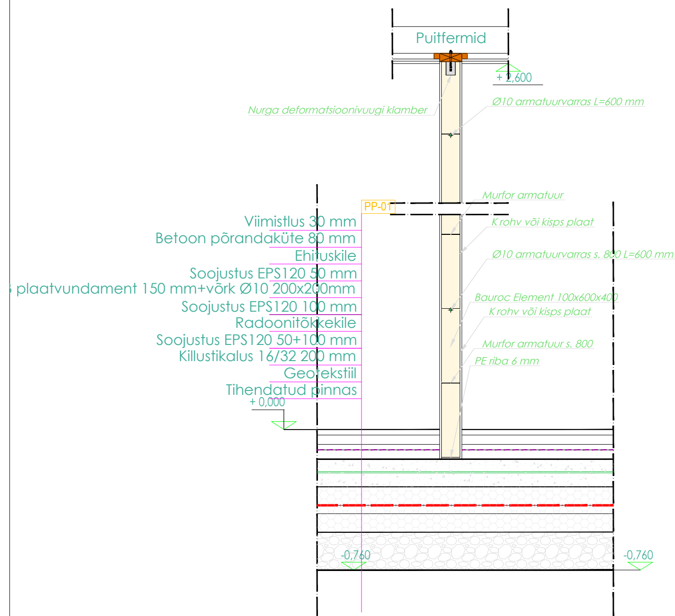
Vertikaalne lõige siseseinad
