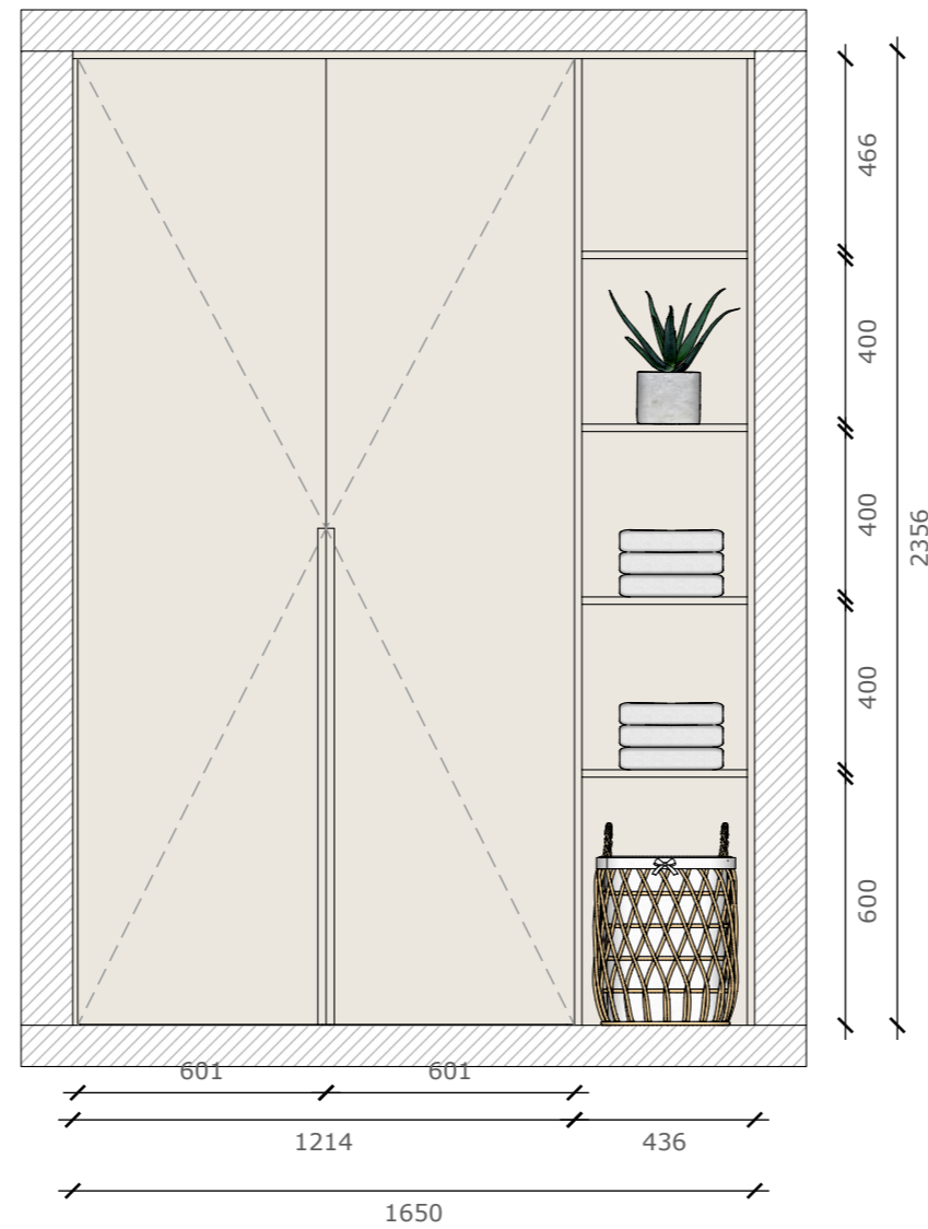
2D OTSEVAADE USTEGA
