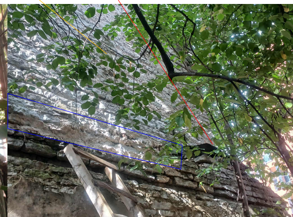
Keskelt on näha värske lõhkumine, kus sideaine (mördi) osa pole veel määratud
