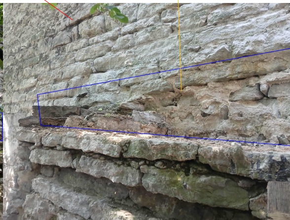
3 ülemist paekivi rida ca 0,5 m pikkust ala on juba ära lõhutud, lõhutud osas on tekkinud erinevaid auke kus vesi sisse pääseb
