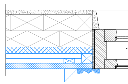
Gaasiseadme suitsutoru kate M 1:10
