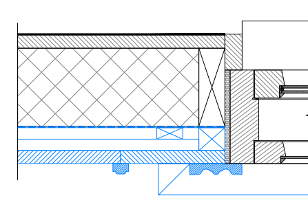
Aknaaluse karniisi pealtvaade sein S-4
