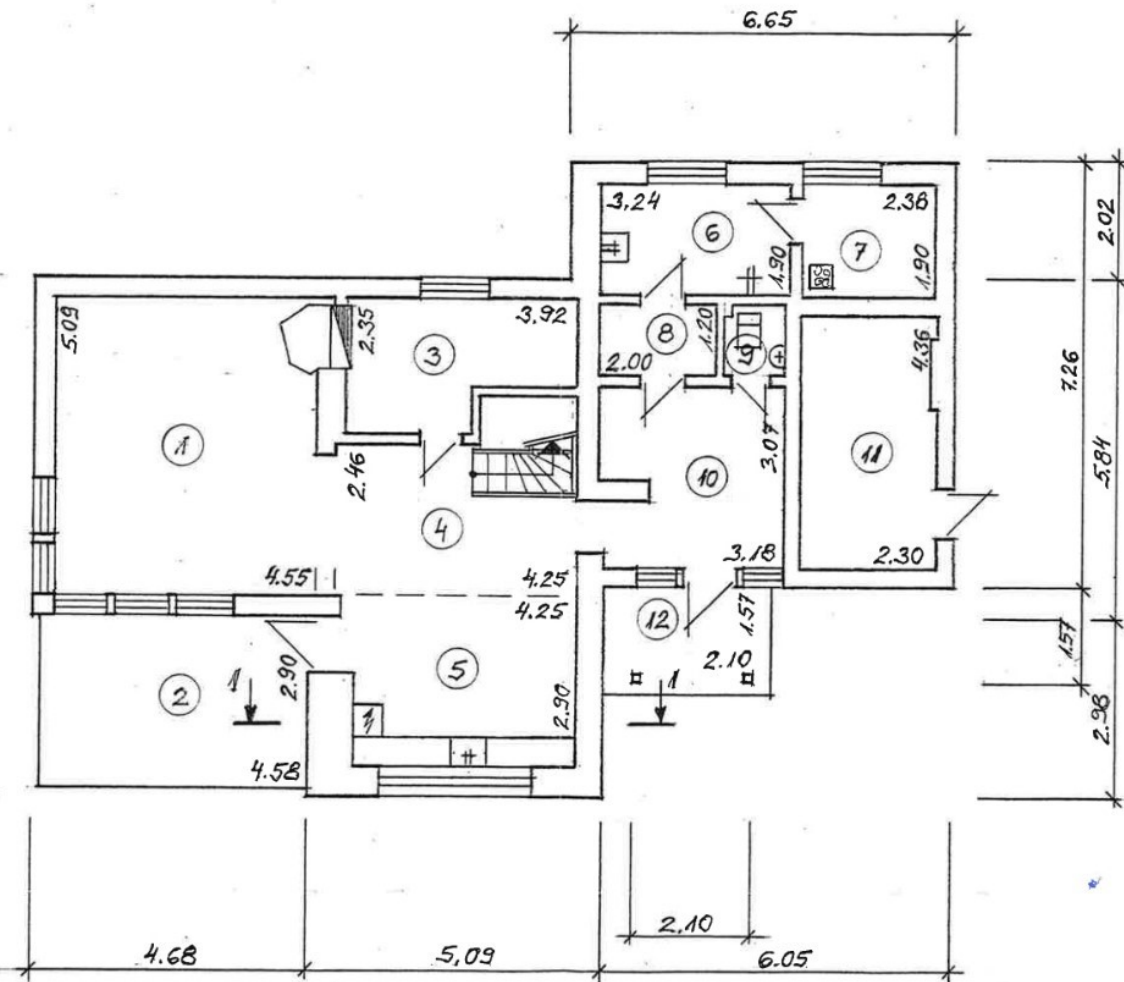
PÕHIPLAAN
