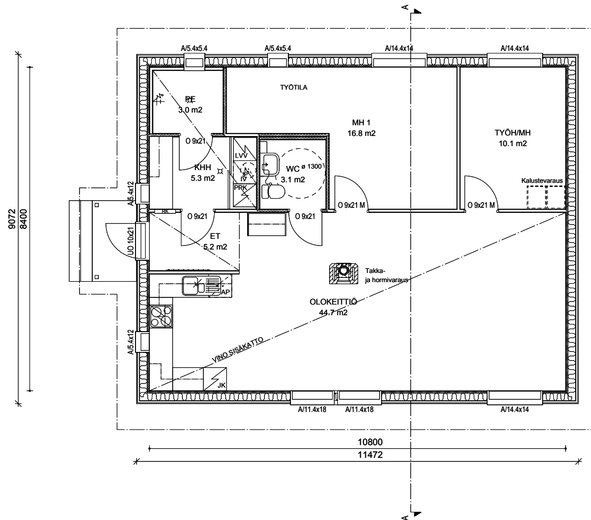
Pohjapiirustus 1.krs
