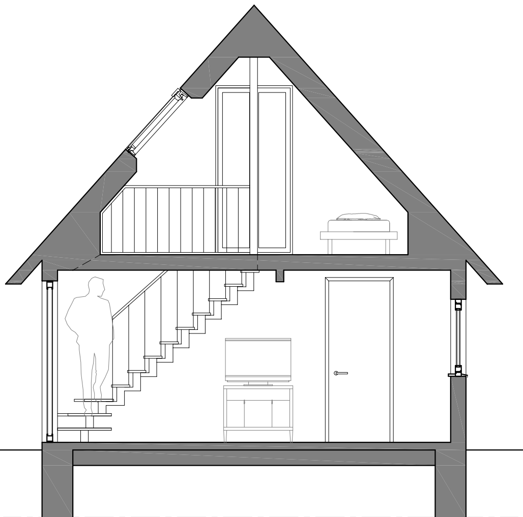
LÕIGE 1-1 M 1:50
