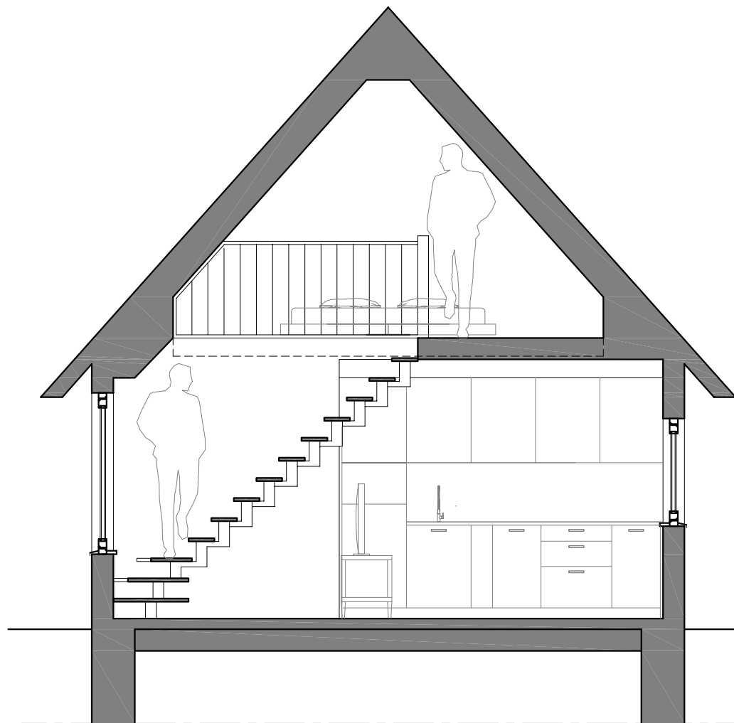
LÕIGE 2-2 M 1:50
