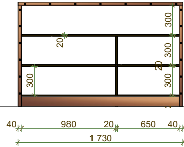
VAADE A mõõtudega
