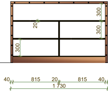
VAADE B mõõtudega
