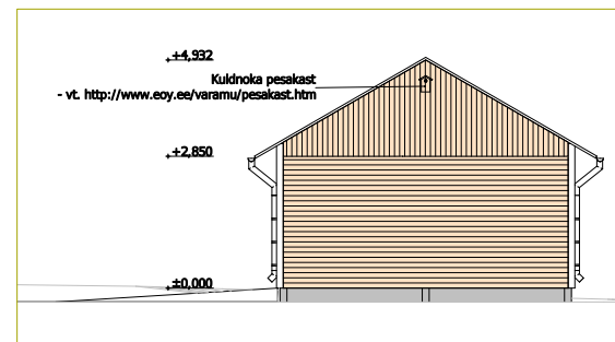
VAADE PAREMALT 1:100
