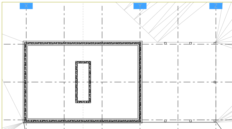
KÕRVALHOONE VUNDAMENDI PLaan 1:100
