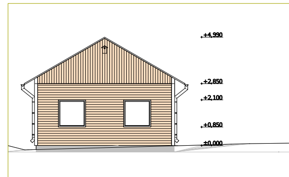
VAADE VASAKULT 1:100
