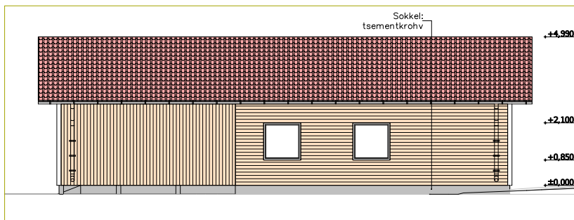
VAADE TAGANT 1:100
