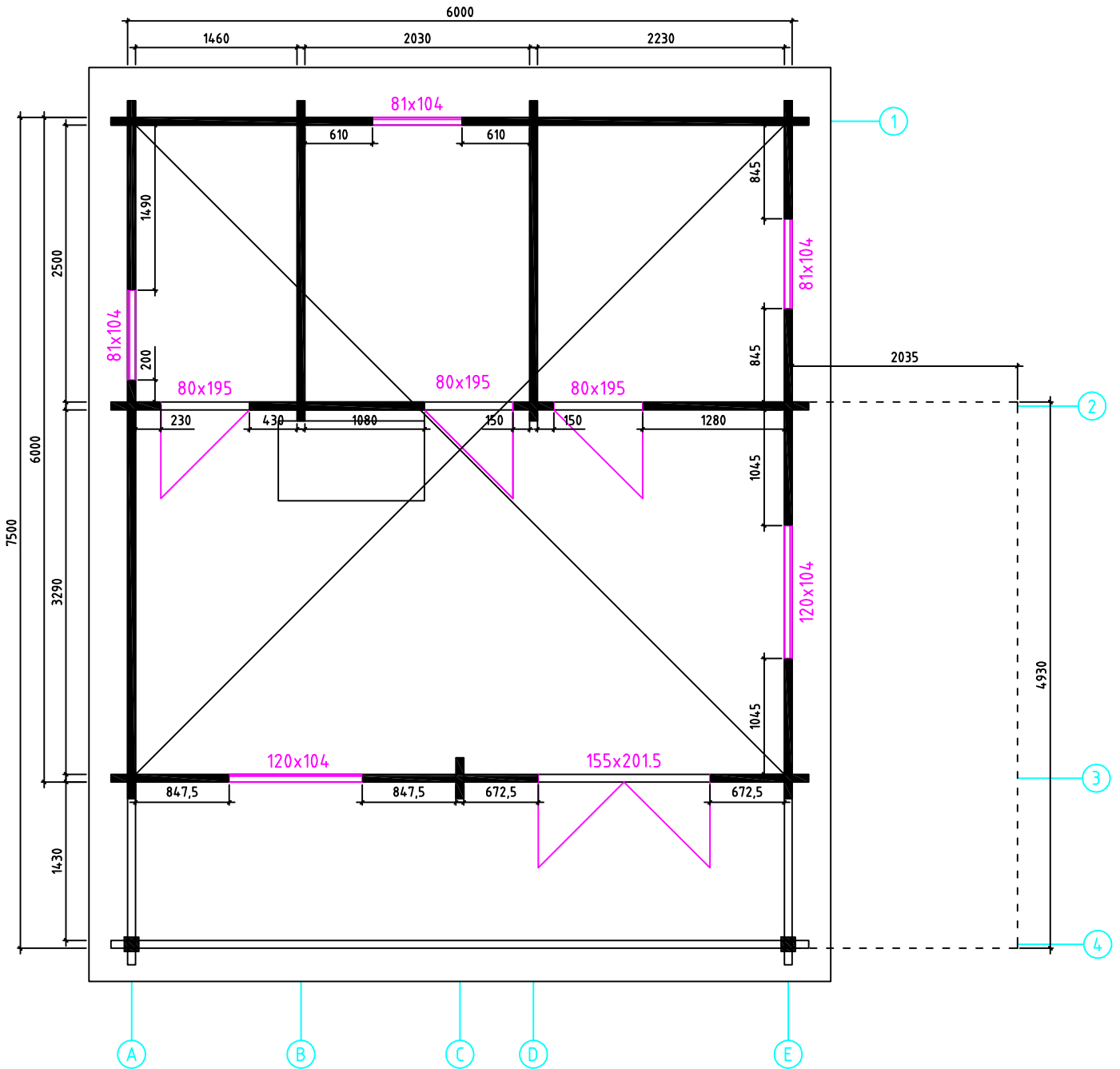
Mari //70/20 Grundplan
