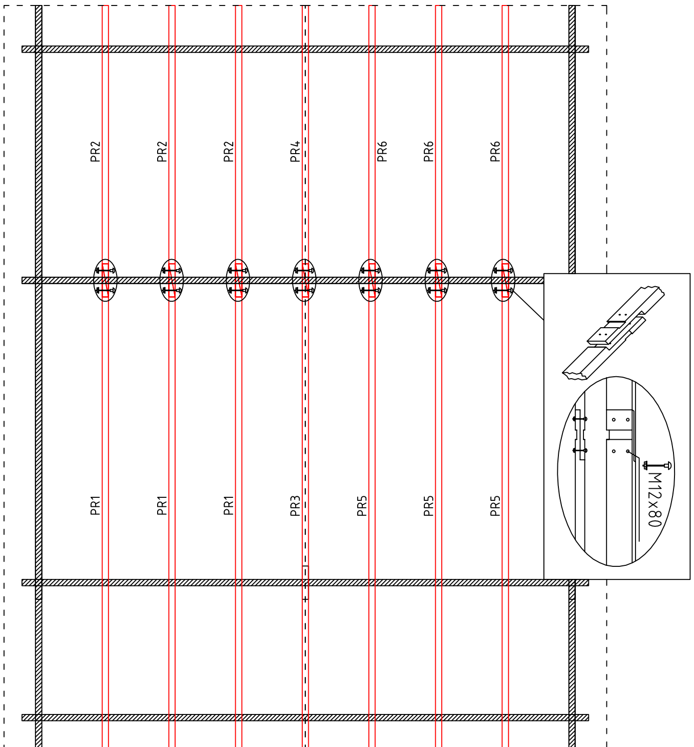
Mari //70/20 Dachbalken
