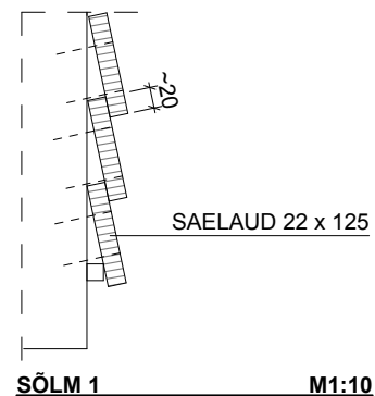
SÕLM 1 M1:10
