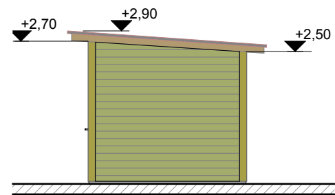
Vaade A 1:100
