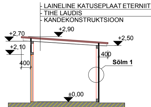
Lõige1-1 1:100
