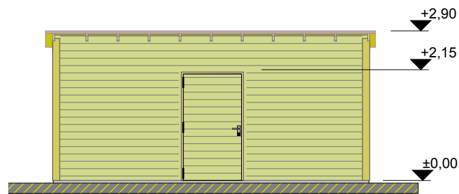
Vaade B 1:100
