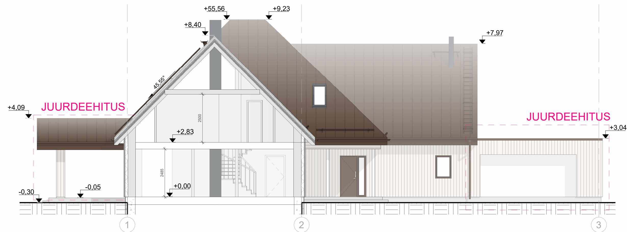
Lõige 1 1 : 100
