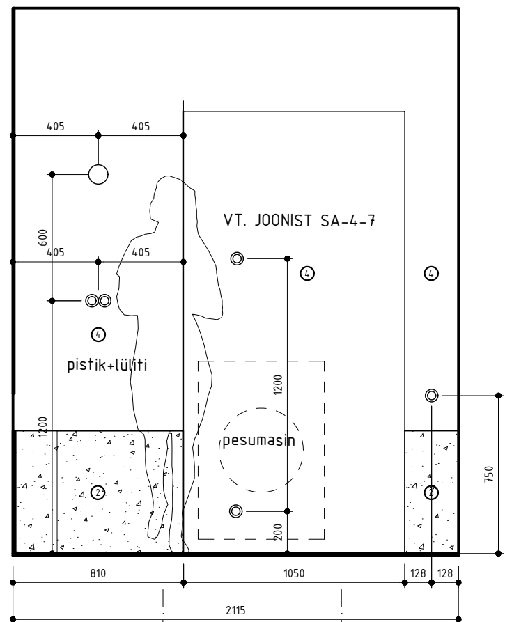
VADE A-A
