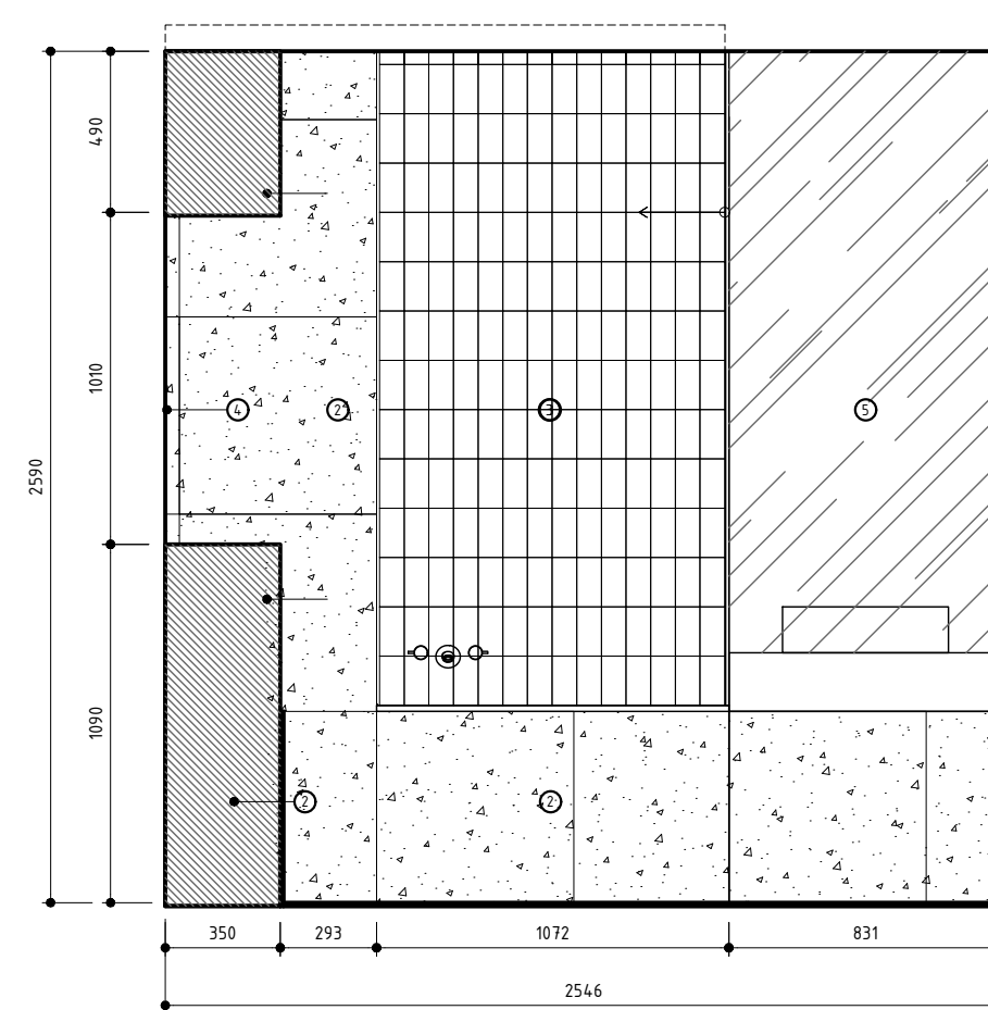
VAADE E-E
