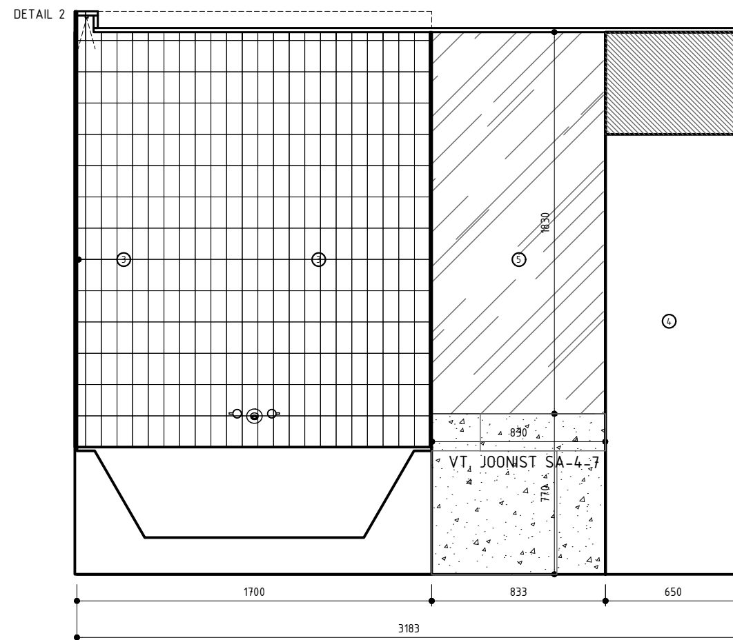
VAADE C-C
