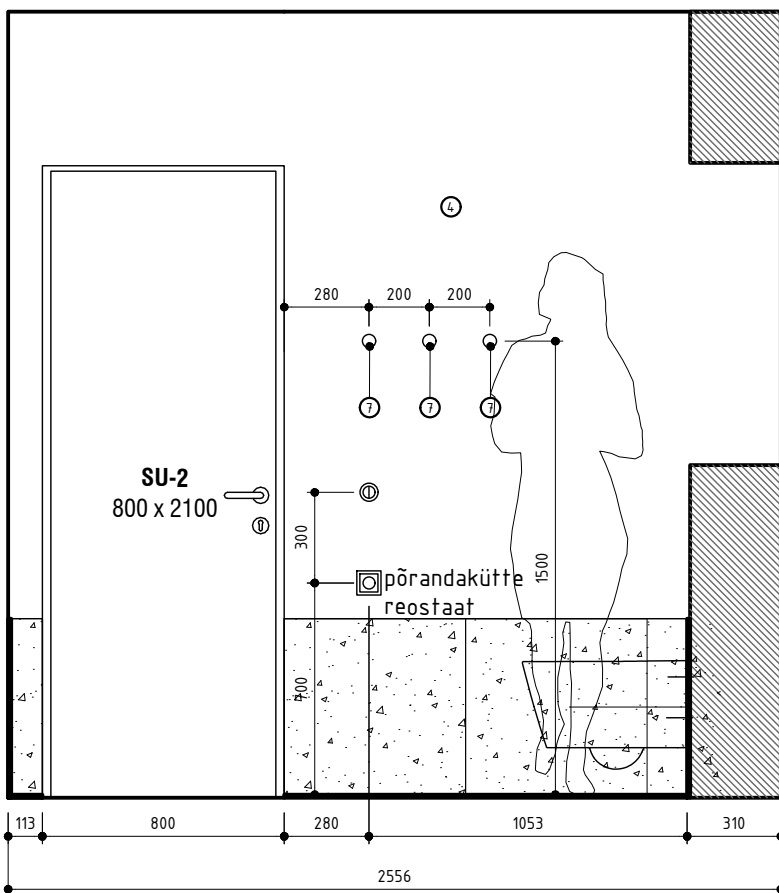
VAADE D-D
