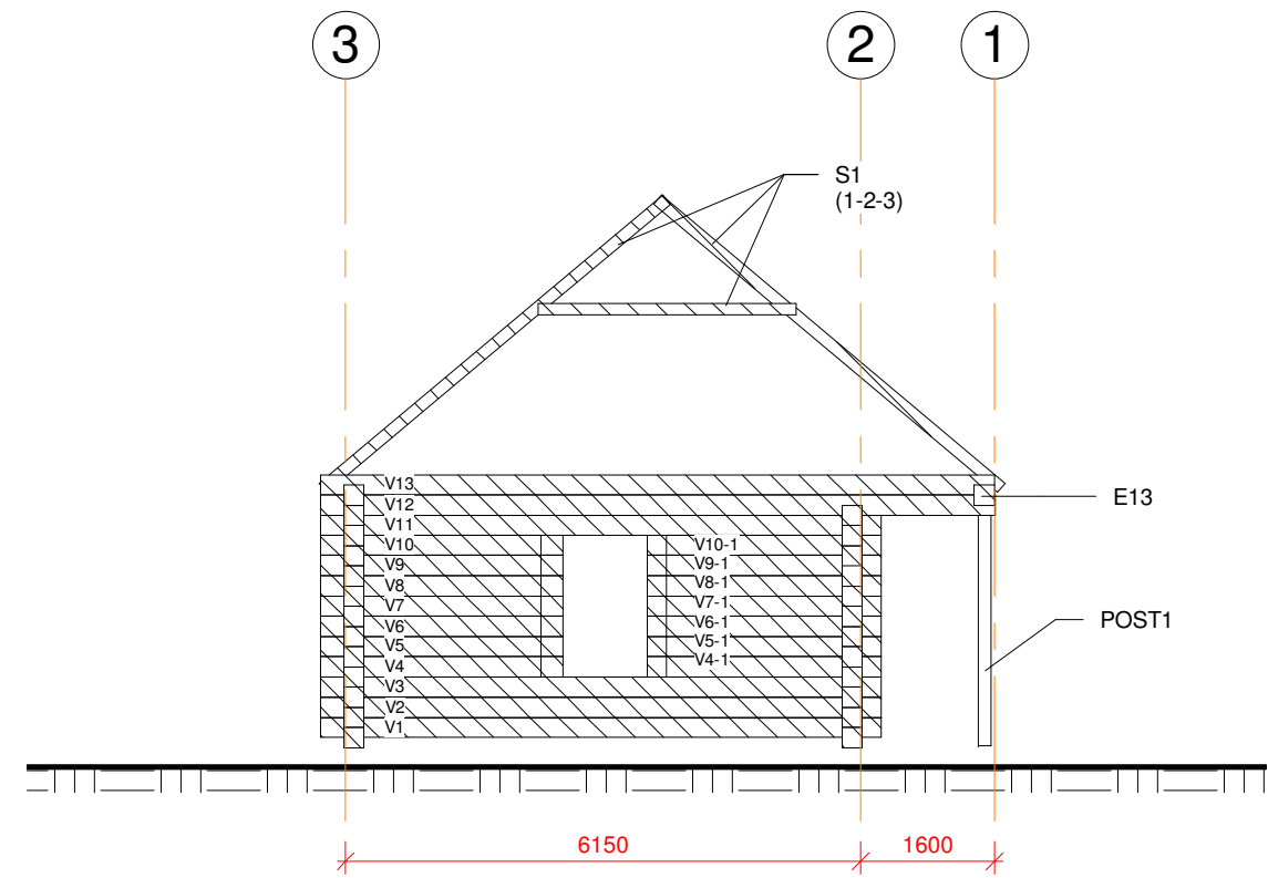
3-1 1 : 100
