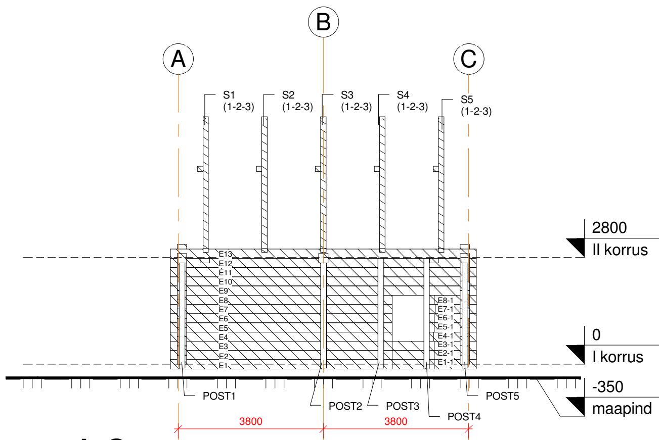
A-C 1 : 100
