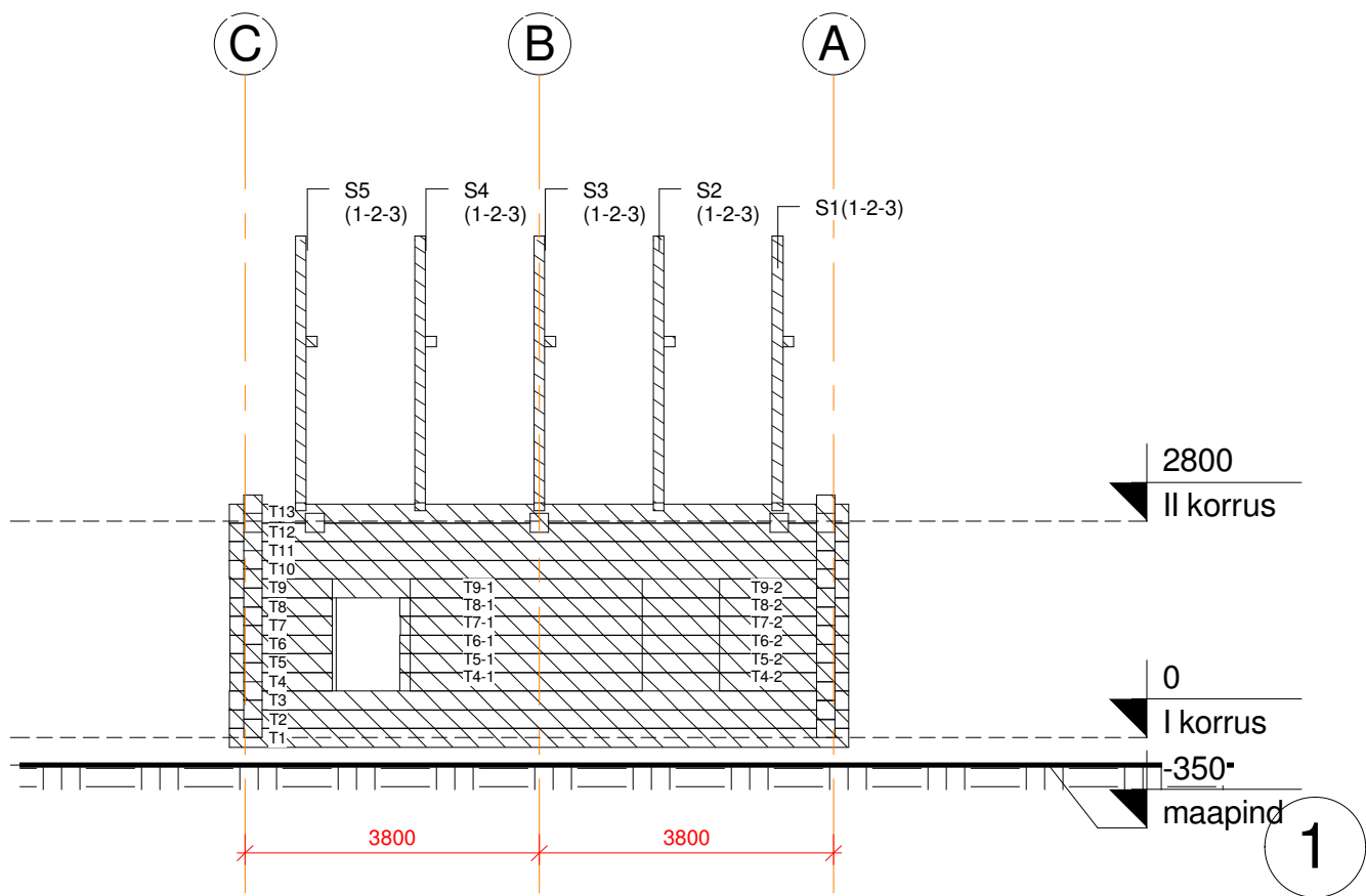
C-A 1 : 100
