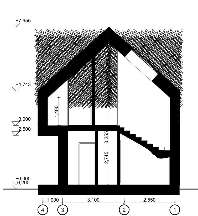
L01 Lõige 1:100
