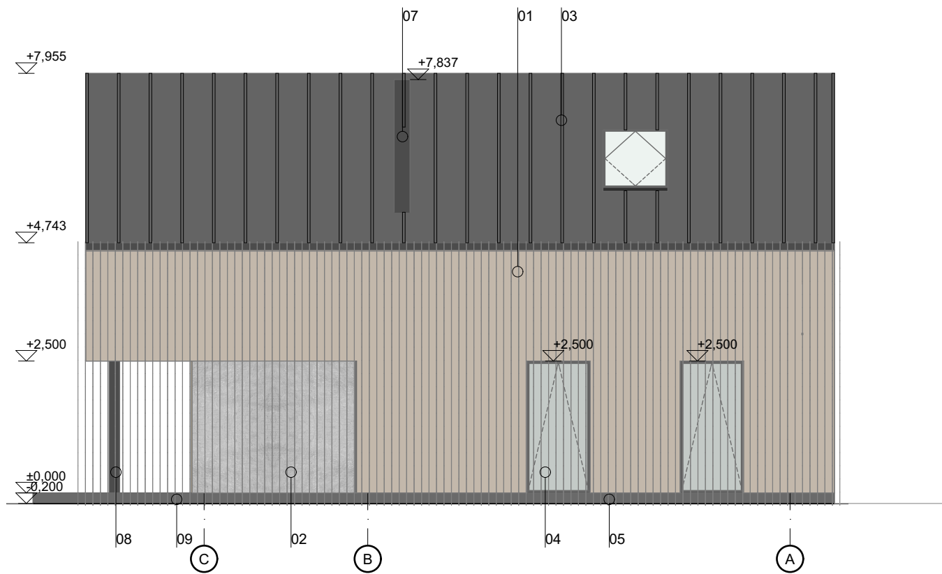
Vaade 2 1:100
