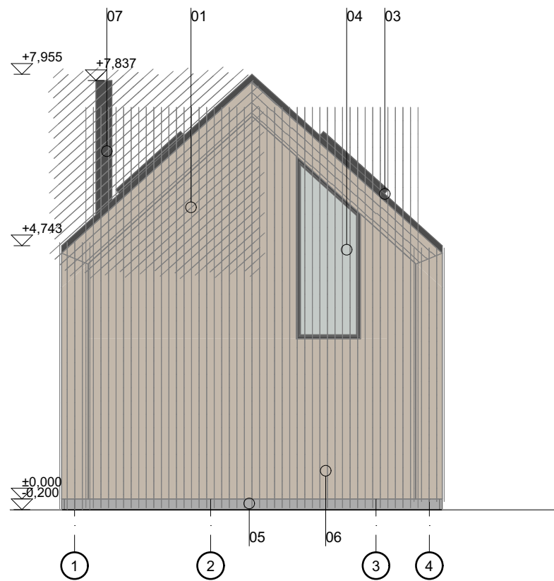
Vaade 1 1:100
