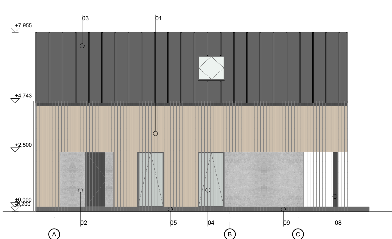
Vaade 4 1:100
