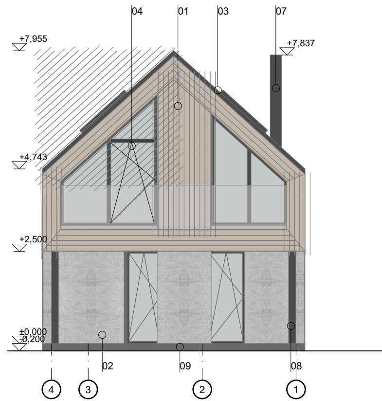
Vaade 3 1:100
