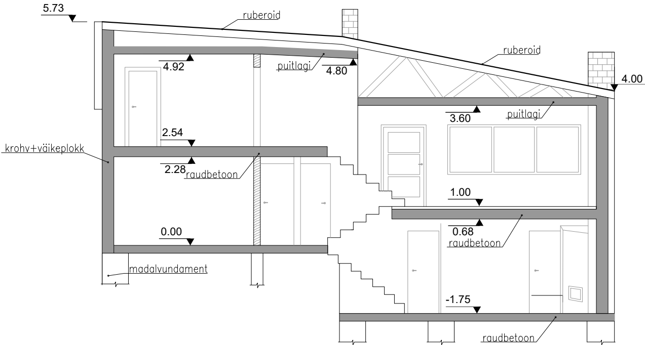
vaade C
