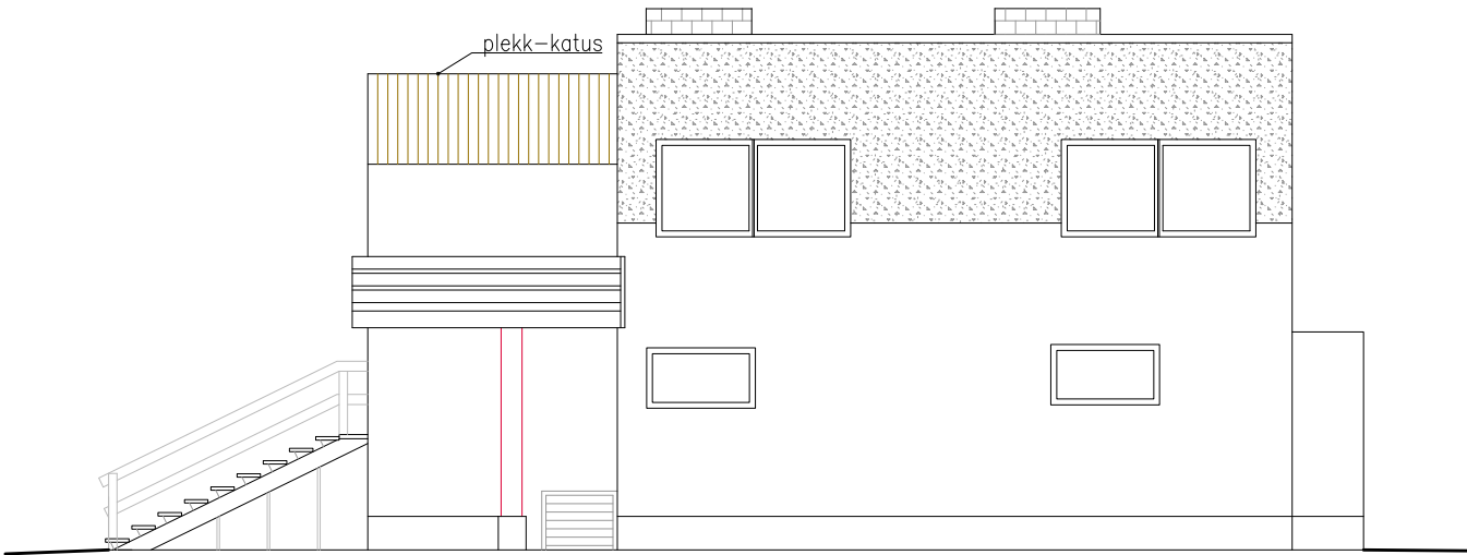
vaade B
