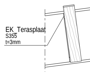
1 - 1 1:10
