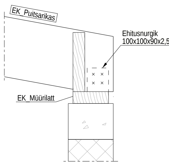
A - A 1:10
