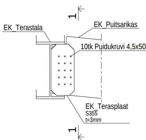
B - B 1:10
