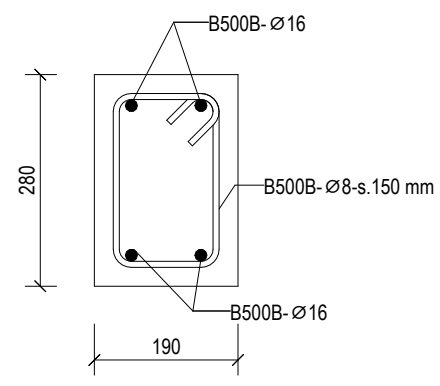
RBL-10 1 : 10
