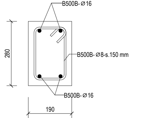
RBL-11 1 : 10
