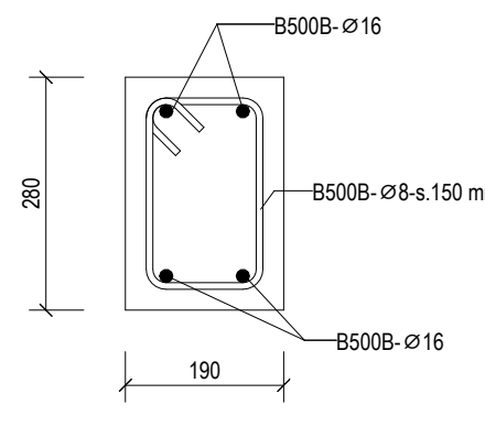
RBL-12 1 : 10
