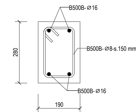
RBL-09 1 : 10
