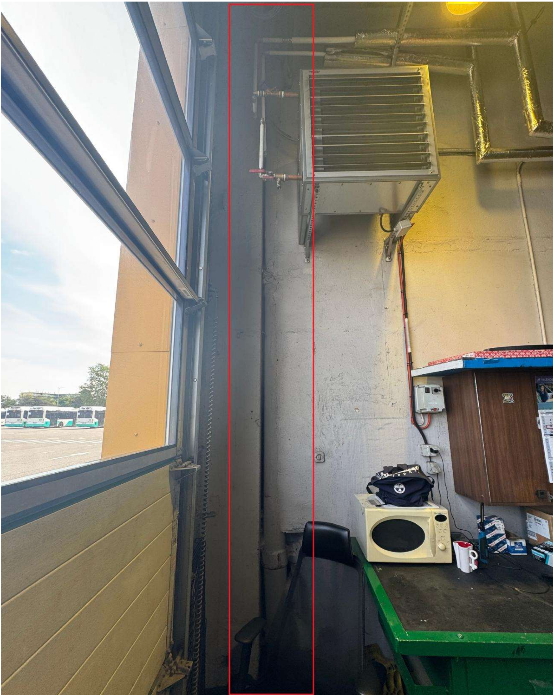
Foto nr 8: Fotel on kujutatud sadaveekanalisatsiooni püstak, mis kuulub rekonstrueerimisele.
