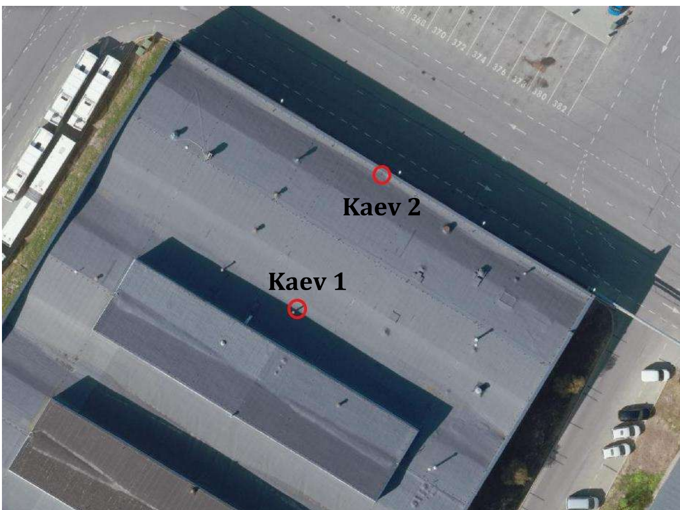
Foto nr 5: Fotel on kujutatud sadeveekaevude asukohad hoone katusel, mille vaheline hoonesisene sadeveekanalisatsiooni torustik kuulub rekonstrueerimisele.
