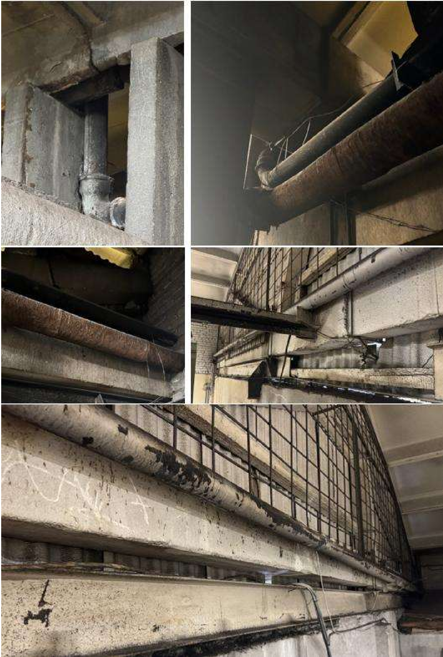
Foto nr 6: Fotel on kujutatud sadeveekaevust 1 alguse saav hoonesisene sadeveekanaliseerimisvõrk, mis kuulub eemaldamisele ning tuleb viia töökoja poolsele seinale.
