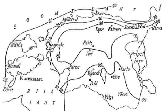
Joonis 5.1 Vihma intensiivsuse q^{20} (l/s*ha) jaotus Eesti territooriumil
