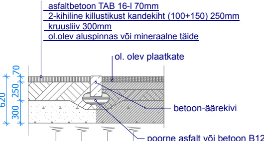
LÕIGE B-B M 1:50
