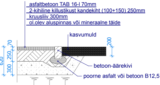
LÕIGE A-A M 1:50
