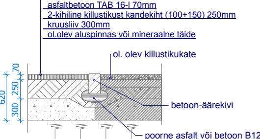
LÕIGE C-C M 1:50
