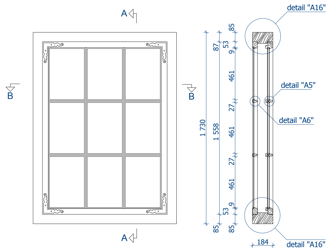
Lõige A - A
