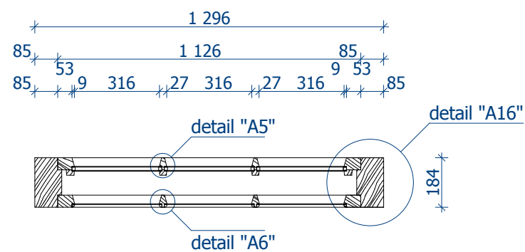
Lõige B - B
