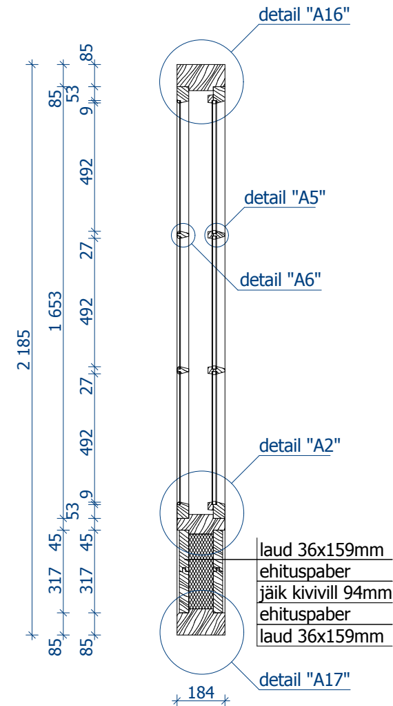
Lõige A - A
