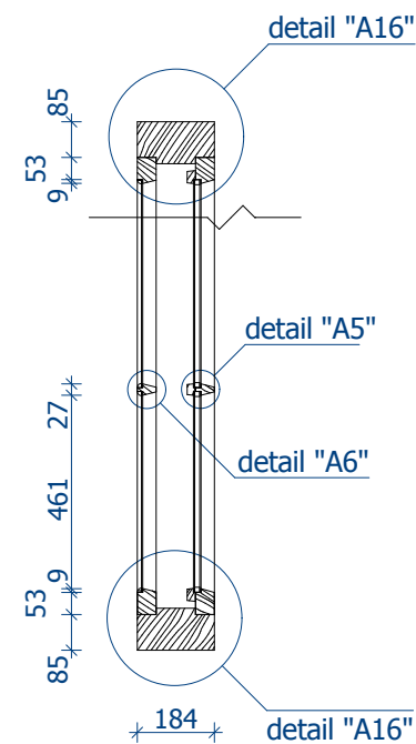
Lõige A - A
