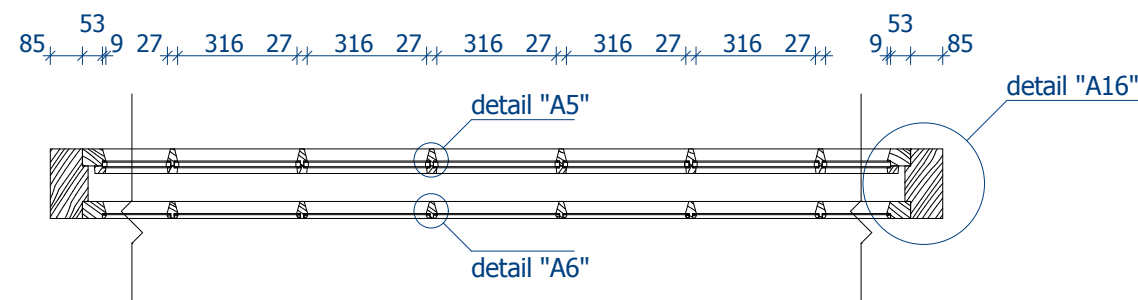
Lõige B - B
