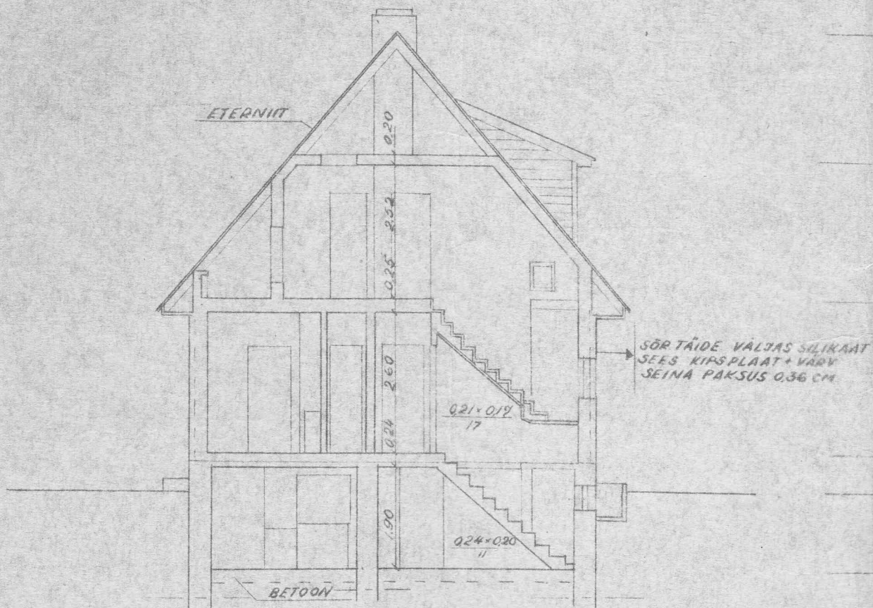
LÕIGE A-A
