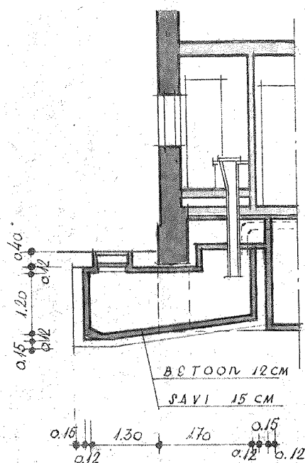
LÕIGES 2-2
