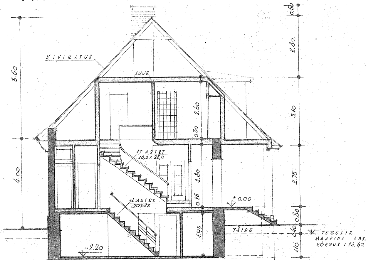
LÕIGES 1-1 1:100
