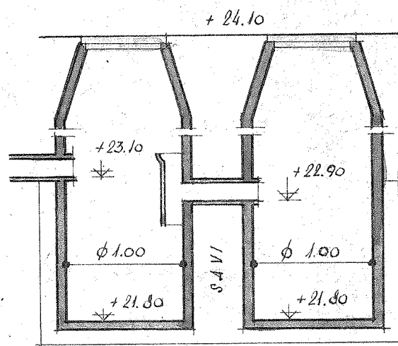
MAJANDUSVEE KOGUMISLAEVUD 1:50
