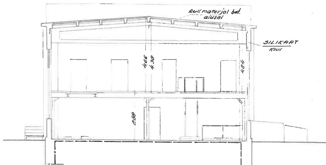
LÕIGE A-A
