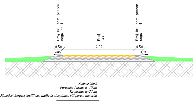
Mahasõidu ristlõige PK 0+20 1:100
