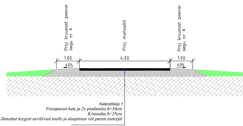
Mahasõidu ristlõige PK 0+05 1:100
