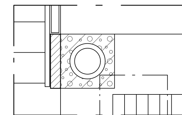
HORMILIITOS 1:20
