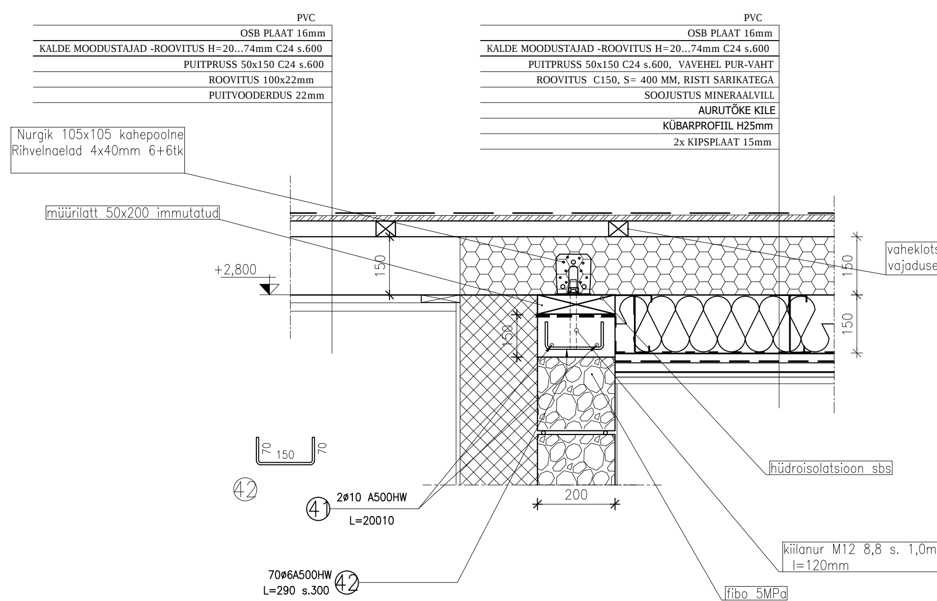
3vk-3vk M1:10
