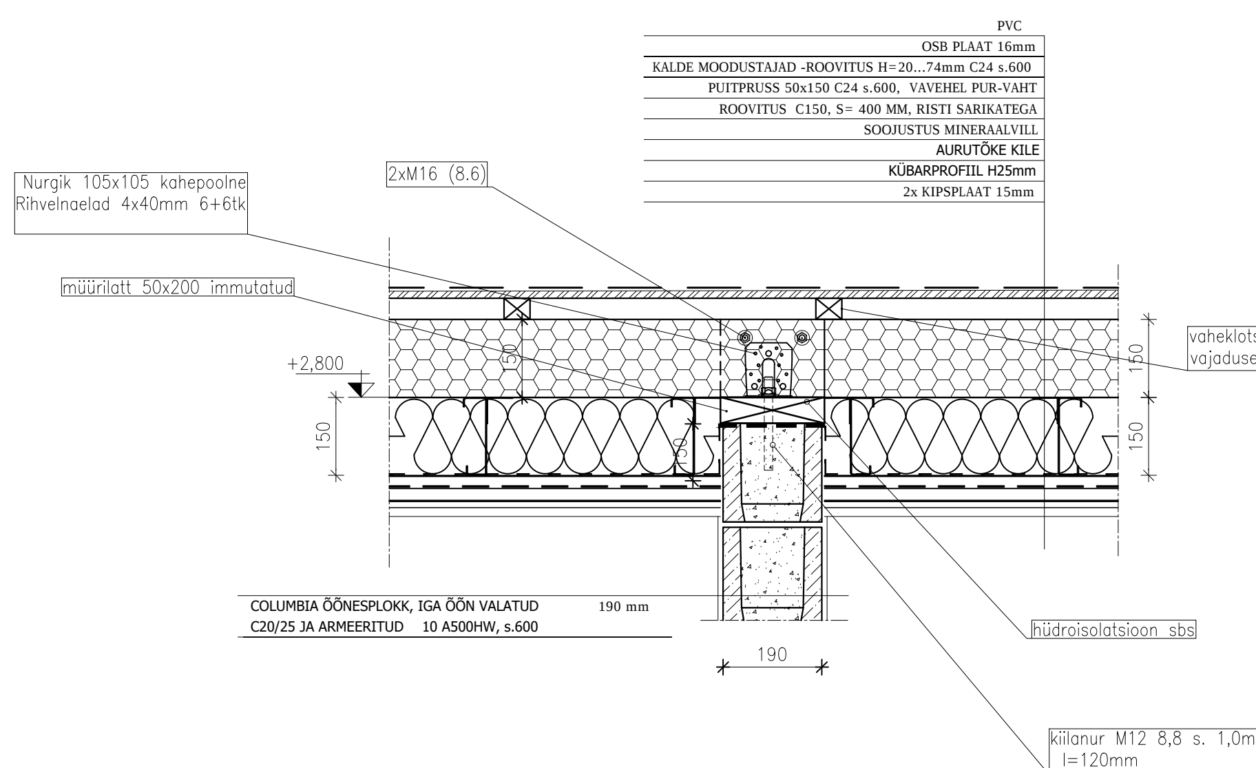
7vk-7vk M1:10
