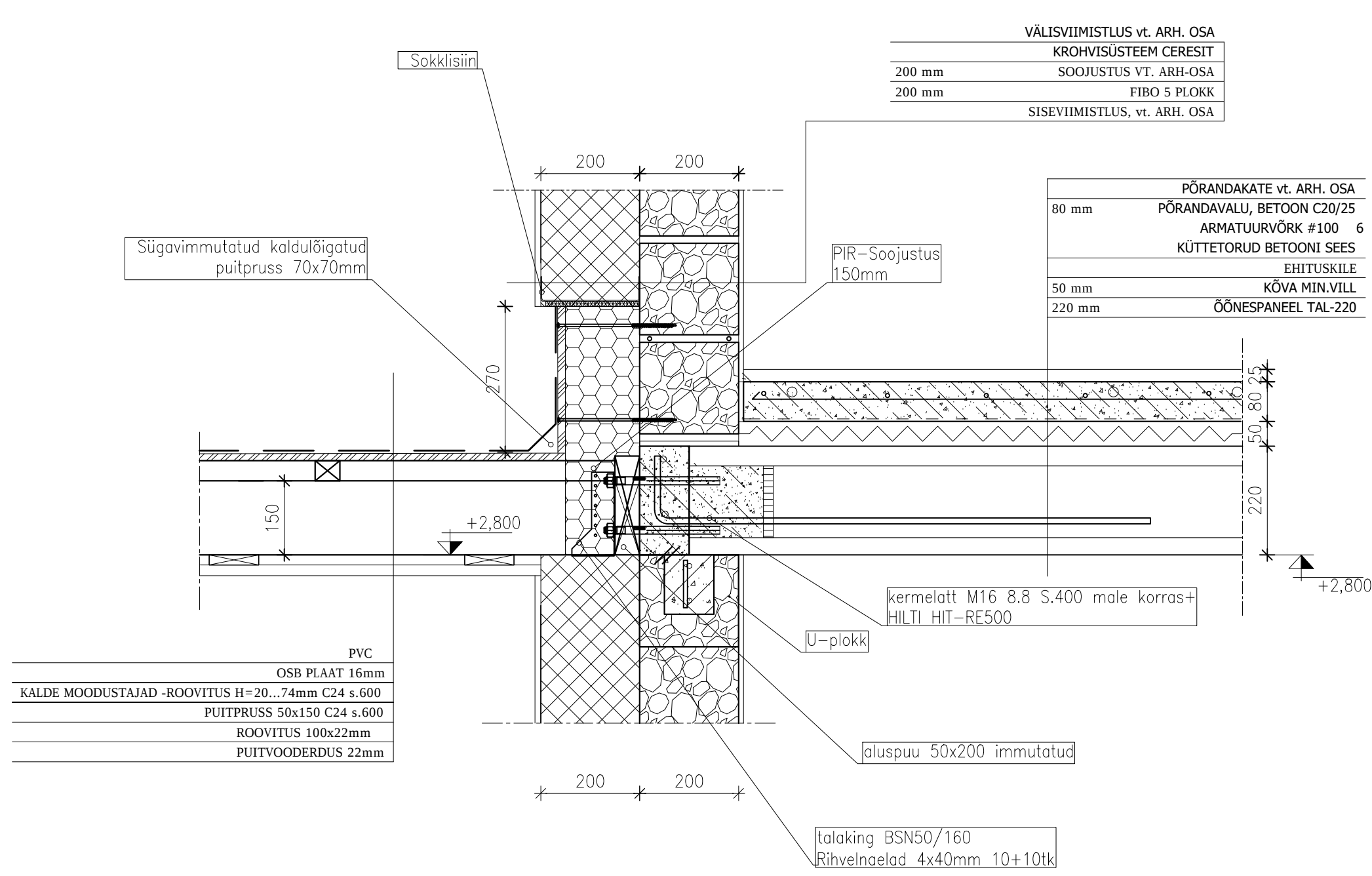
7vk-7vk M1:10
