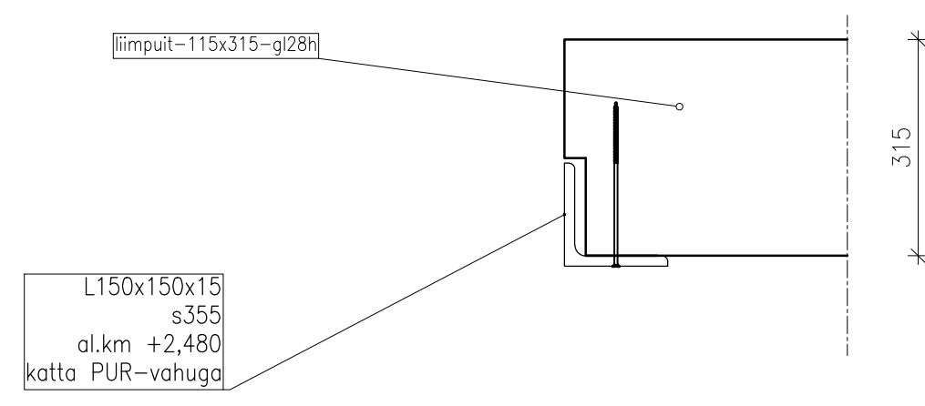
D2 M1:10
