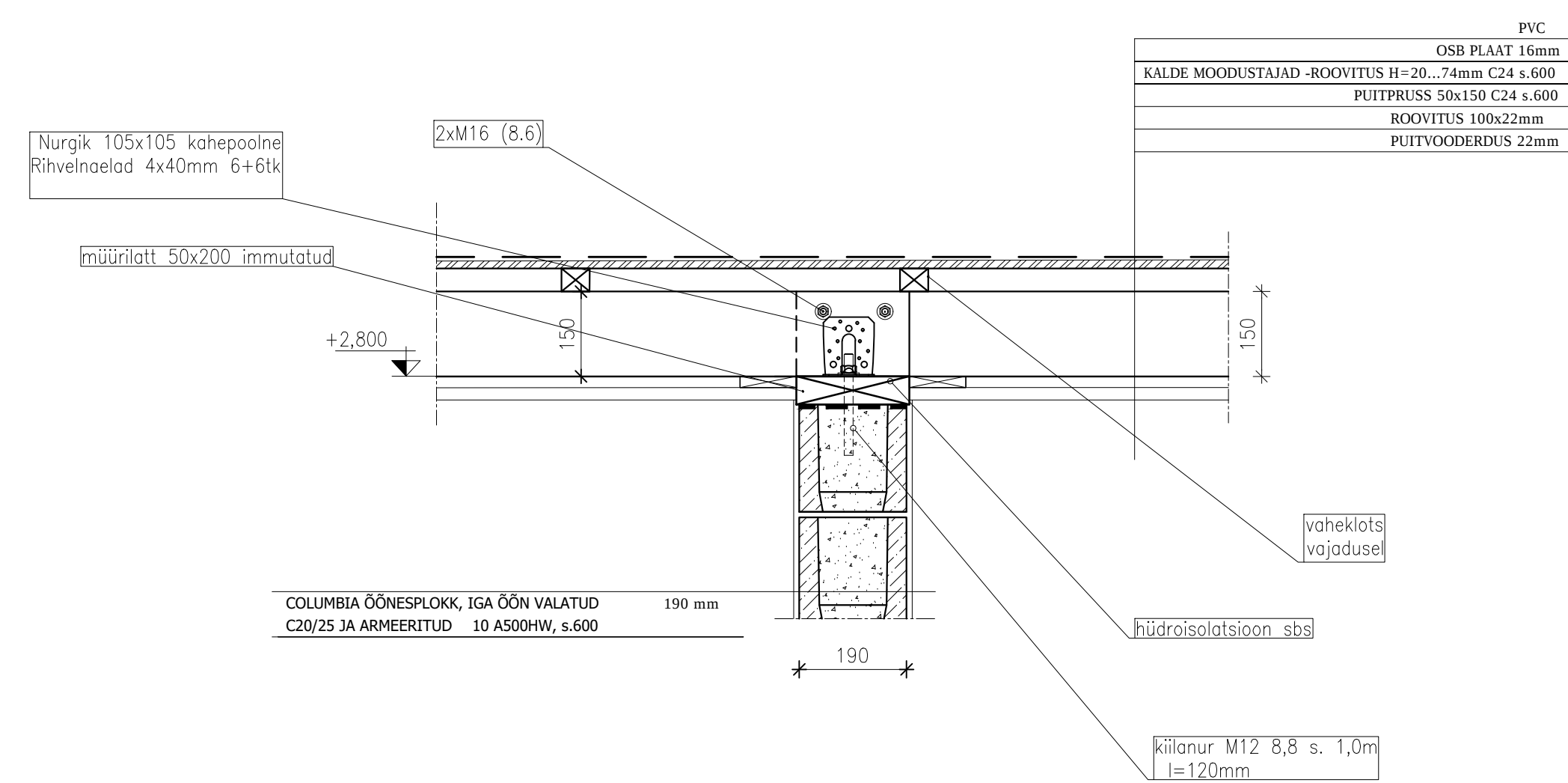
D2 M1:10
