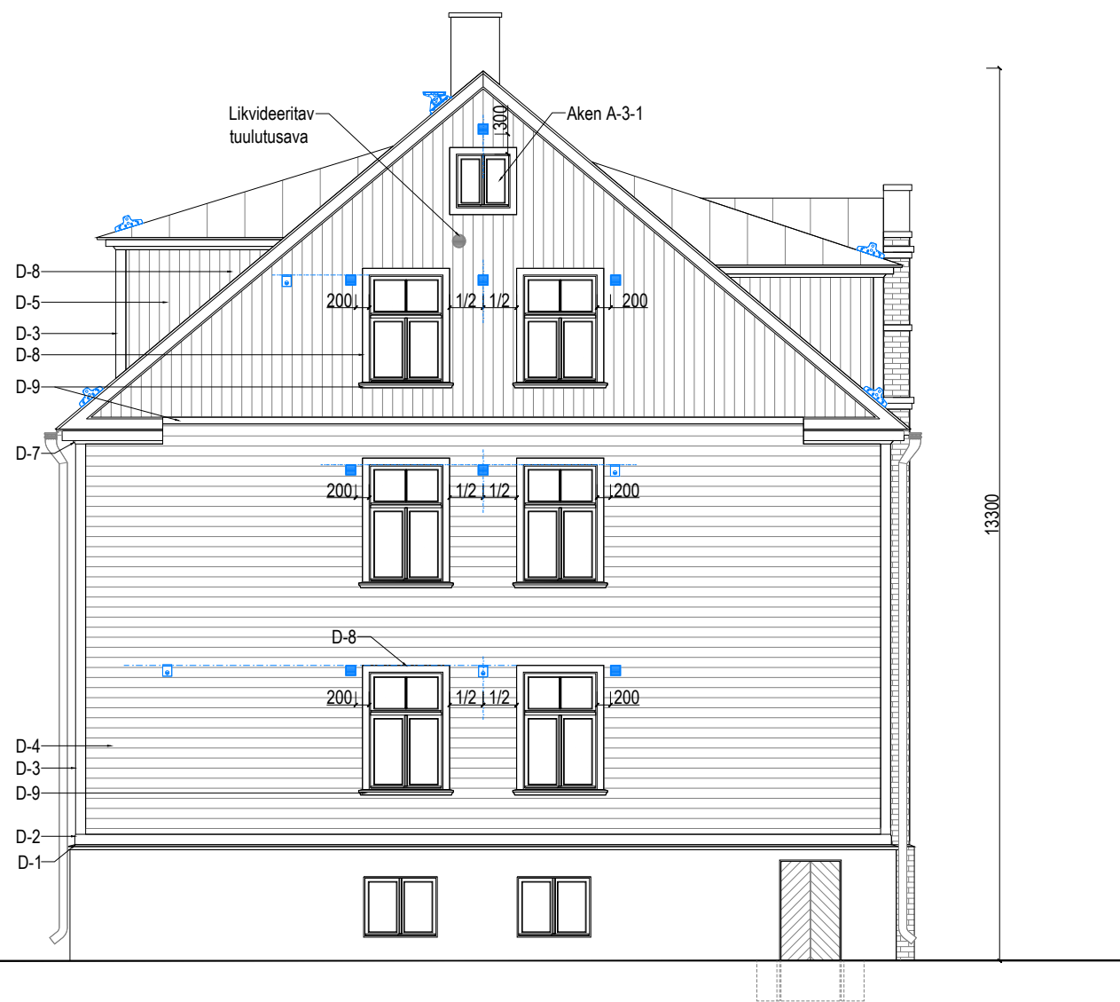
VAADE B
