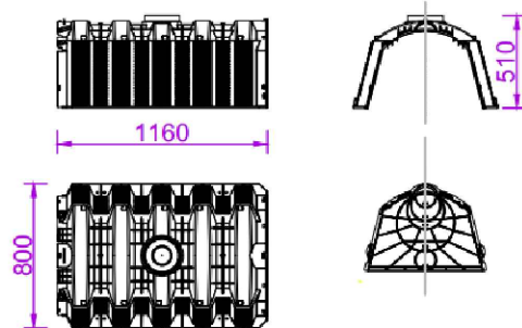
Graf tunnelemendi plaan ja vaated
