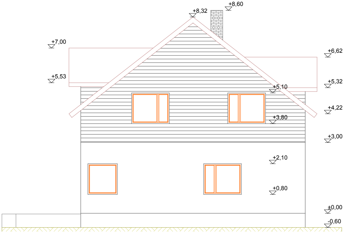
Idast Vaade 1:100
