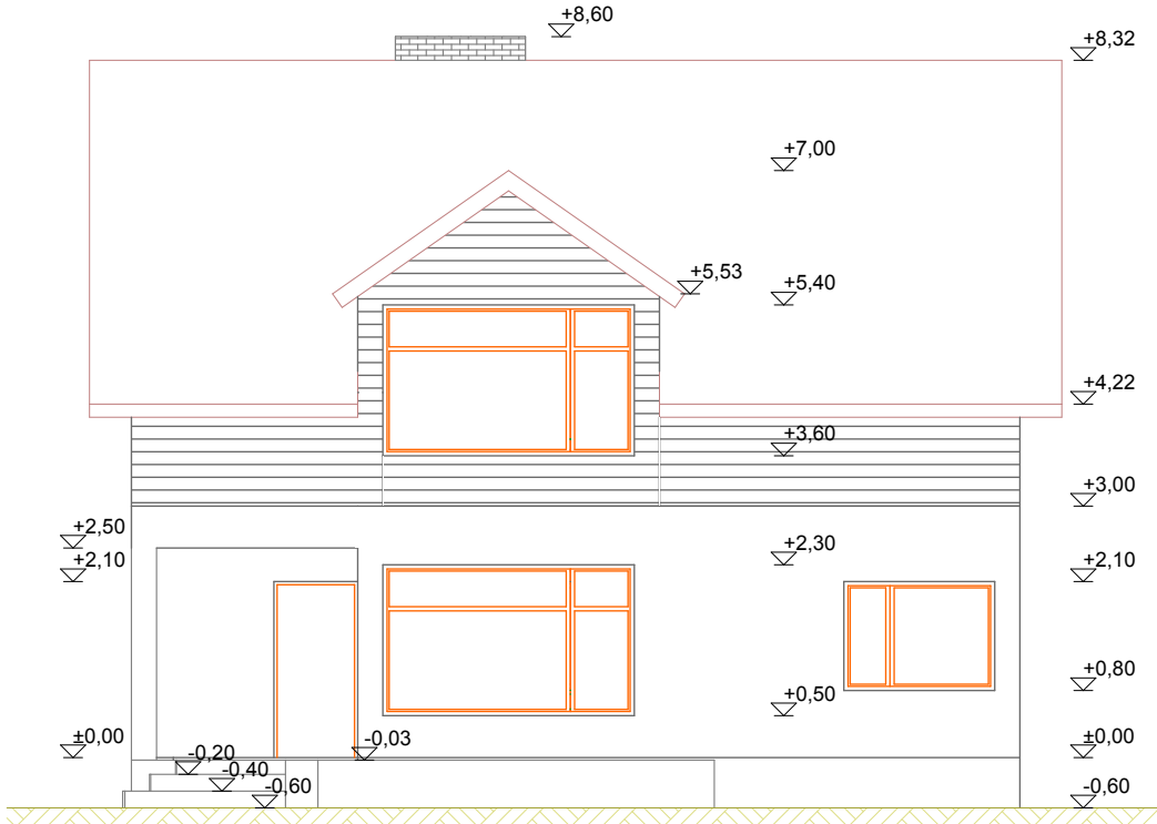
Lõunast Vaade 1:100
