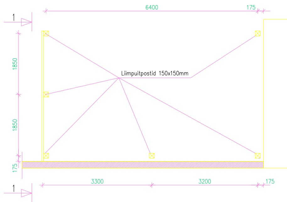
Lõige 1-1
