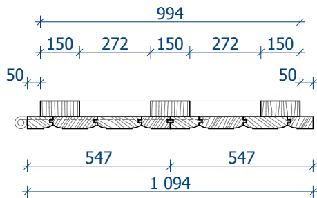
Lõige B-B
