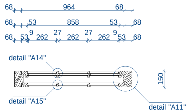
Lõige B - B
