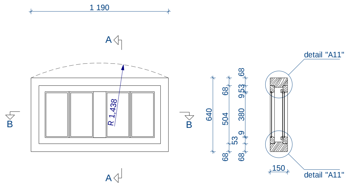
Lõige A - A
