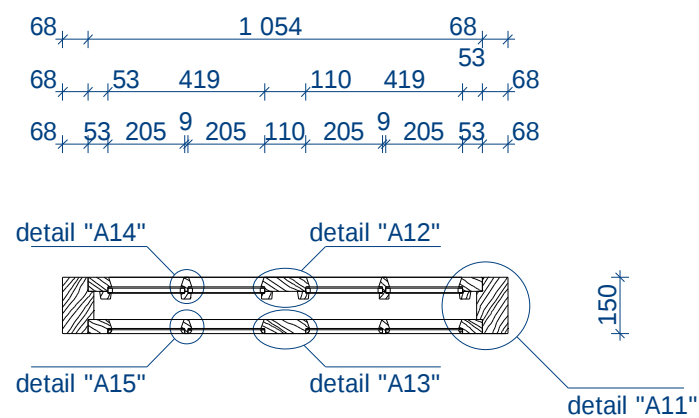
Lõige B - B
