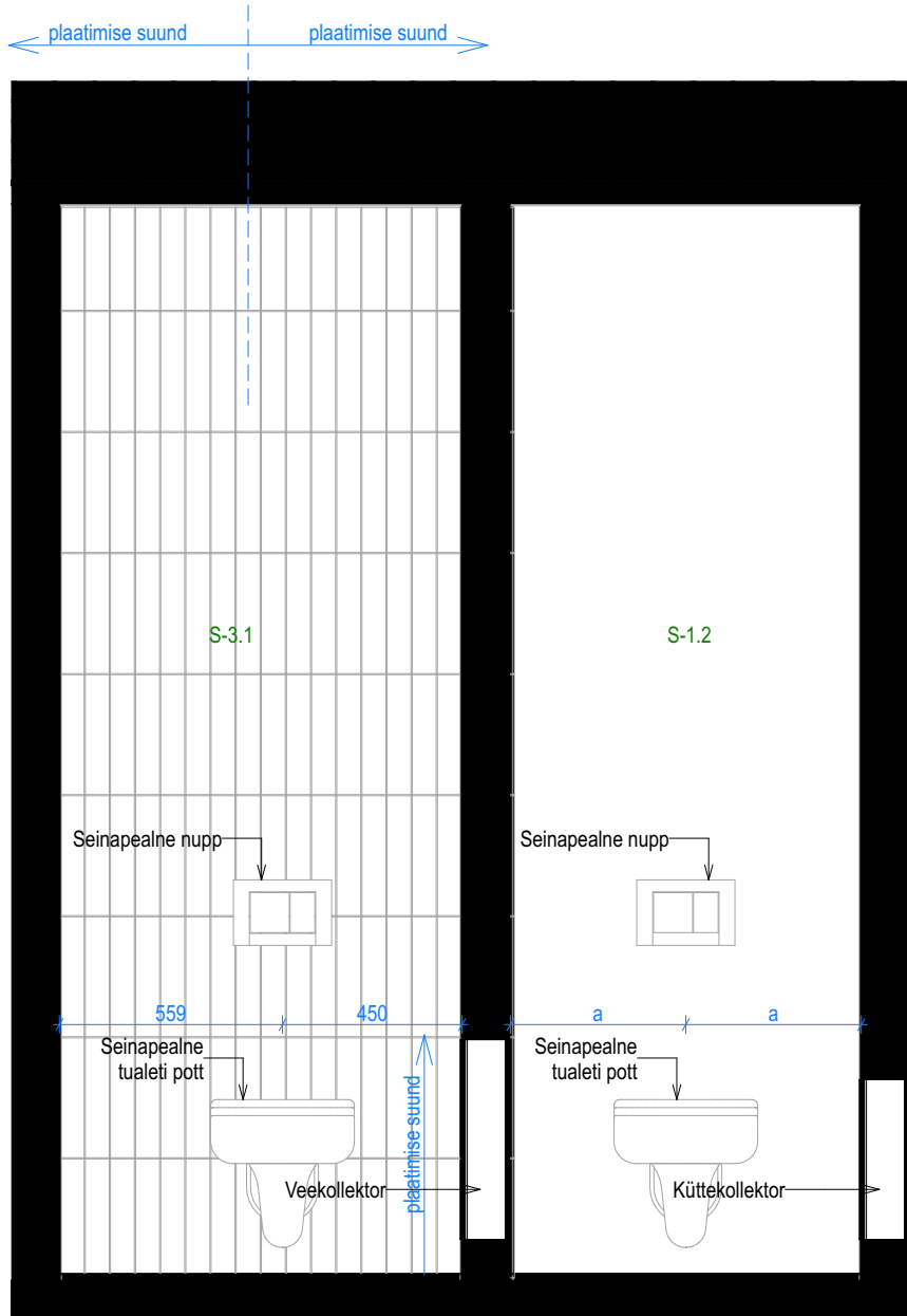
Sisevaade SV05
