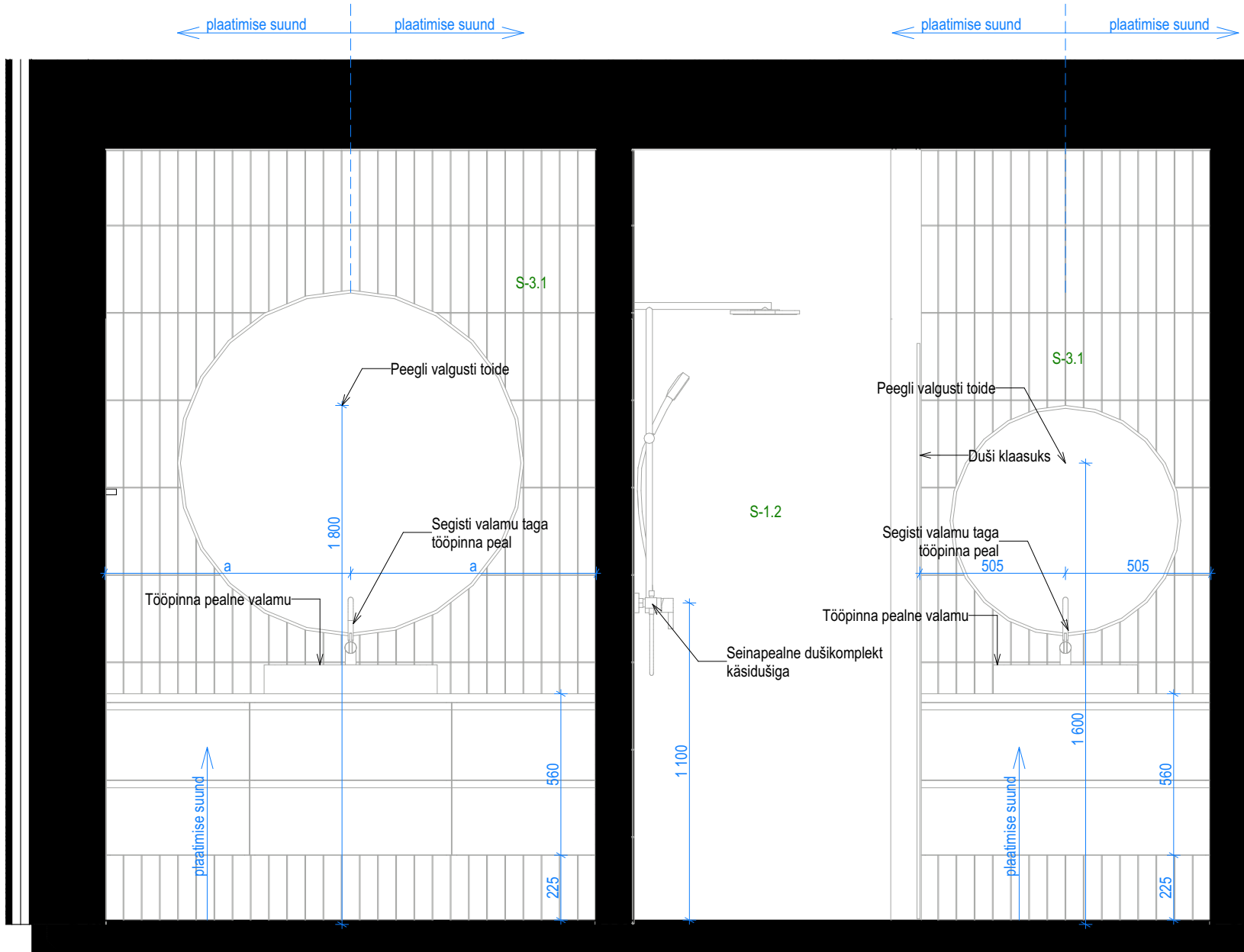
Sisevaade SV01
