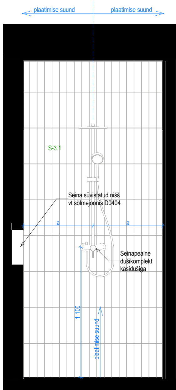
Sisevaade SV06
