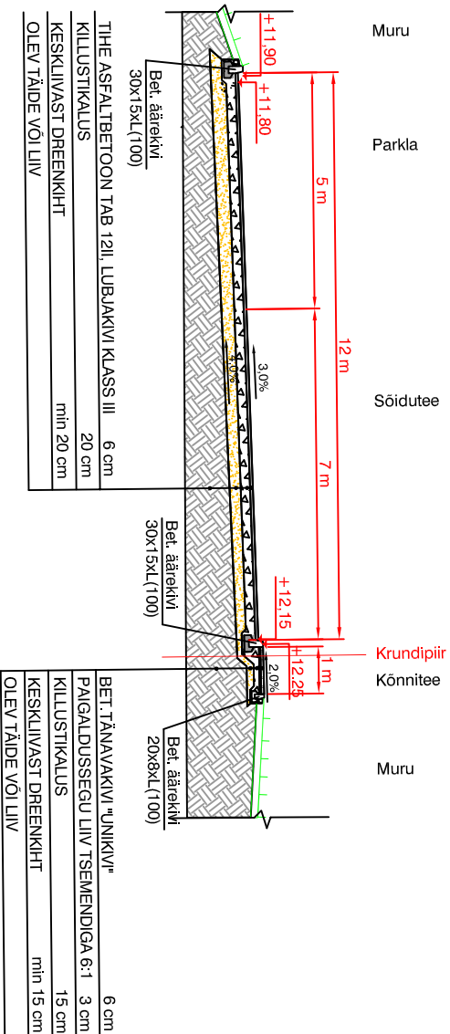
LÕIGE 3-3 M 1:100
