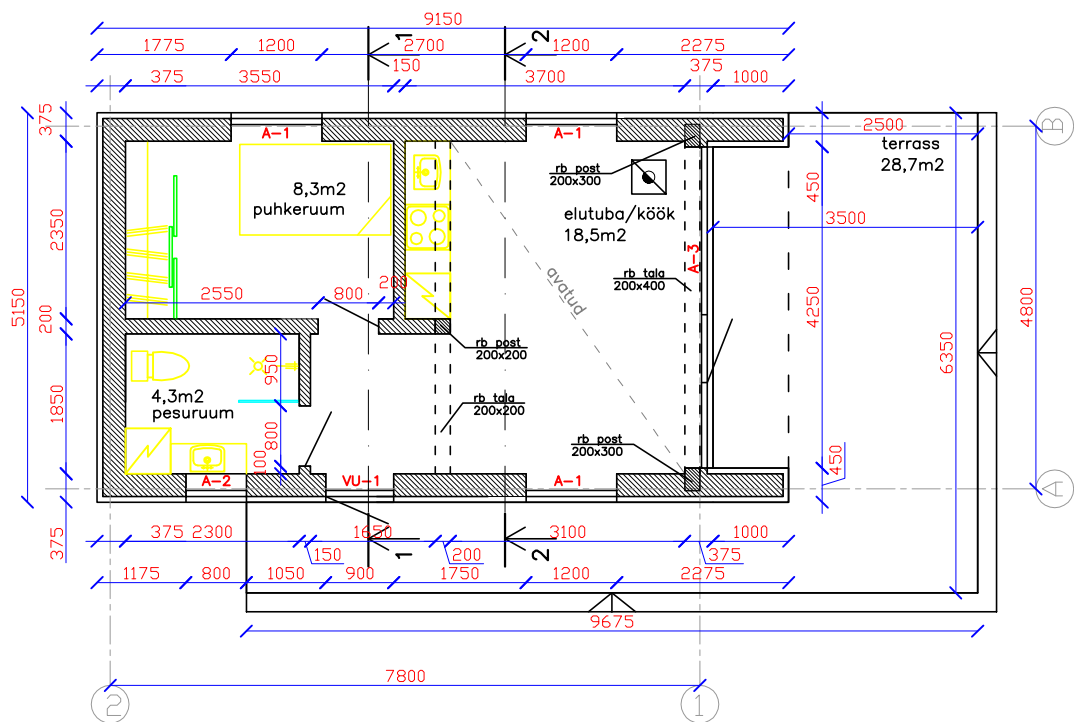
1. korruse plaan
