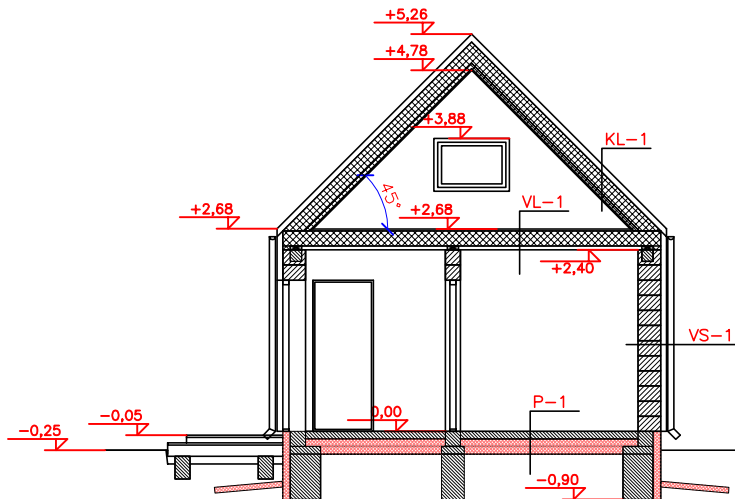
lõige 1-1
