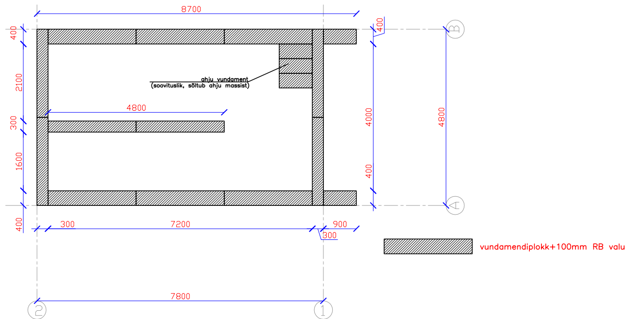
vundamendi plaan
