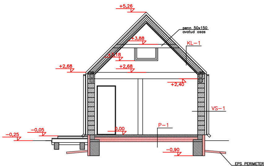
lõige 2-2
