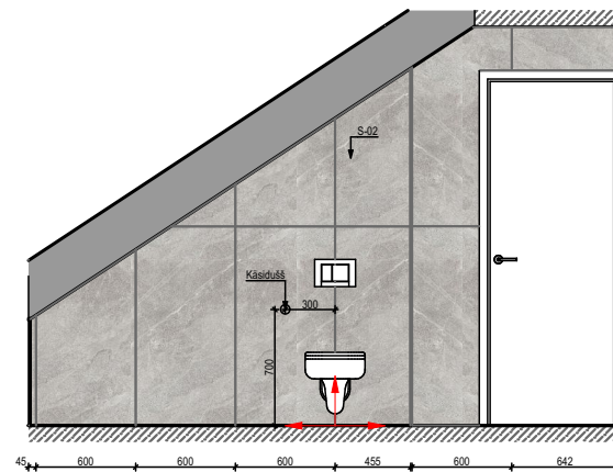
04 1:50
