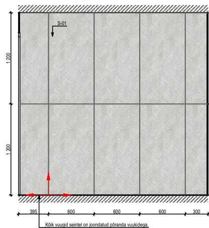
01 1:50
