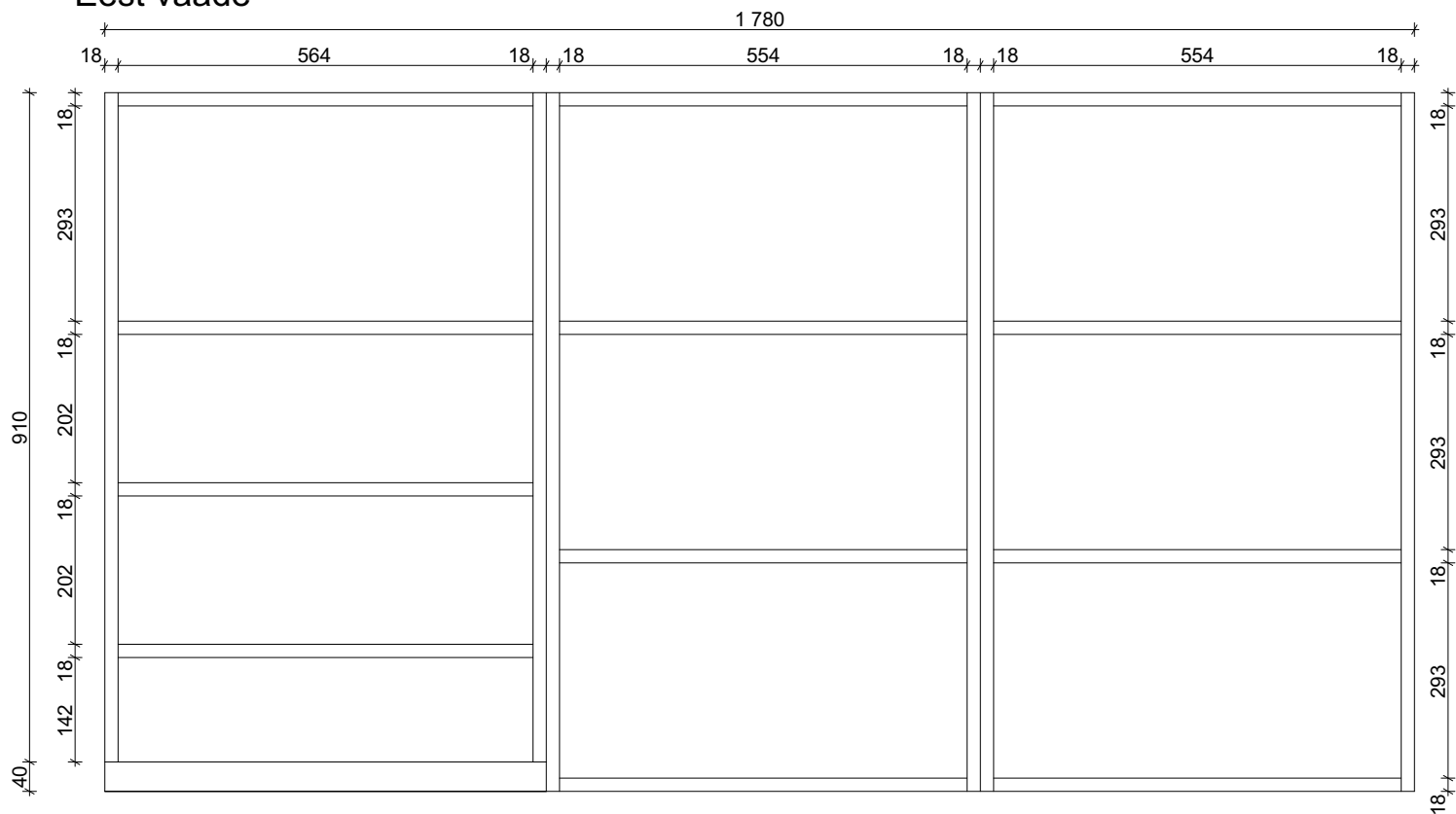
Eest vaade
