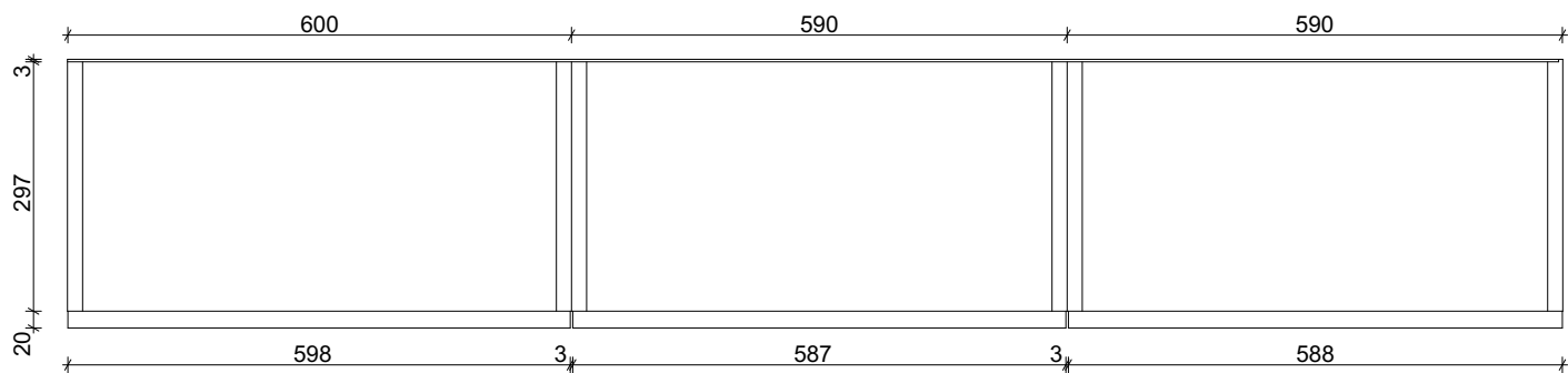
Pealt vaade
