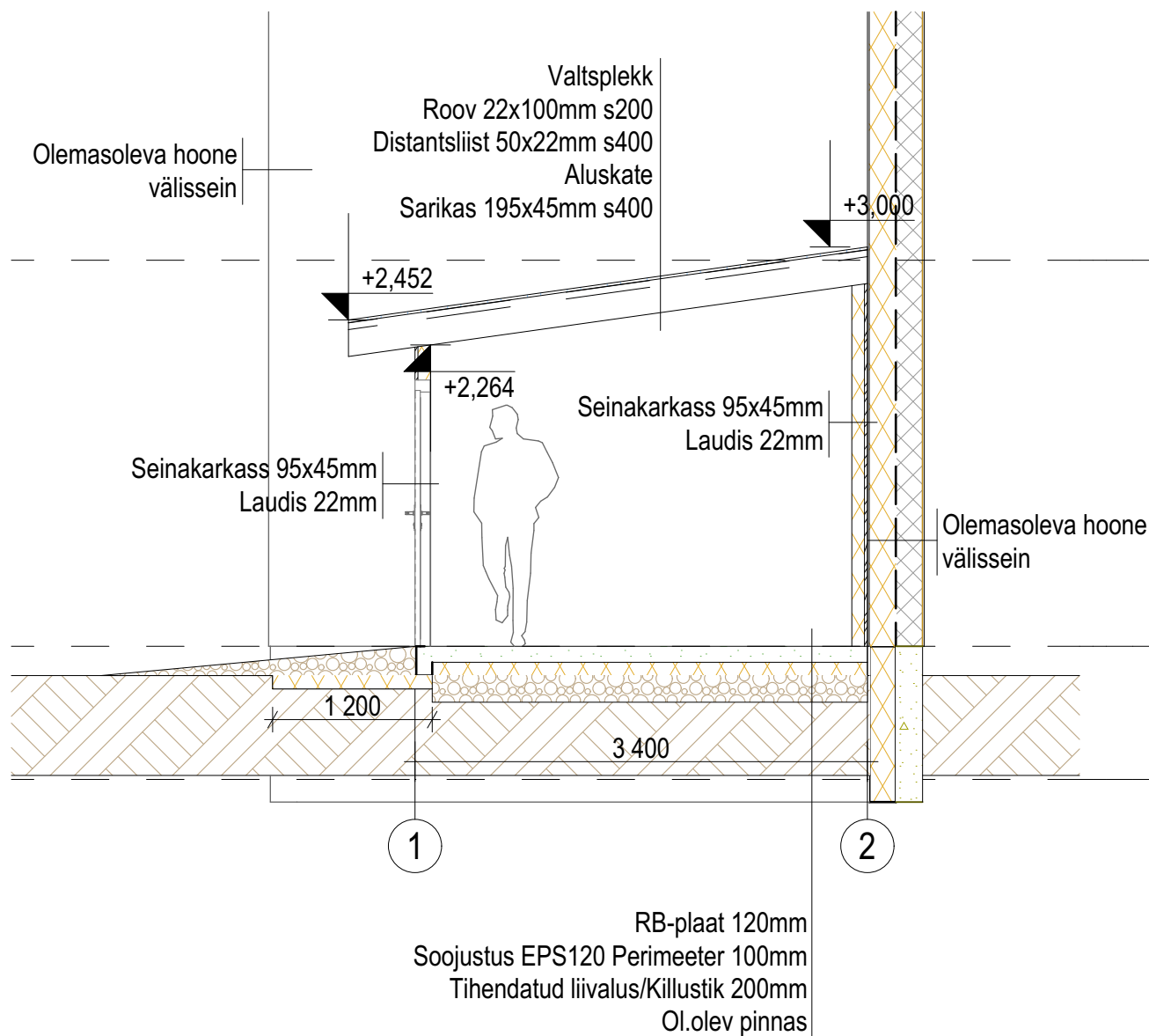
Lõige 1-1
