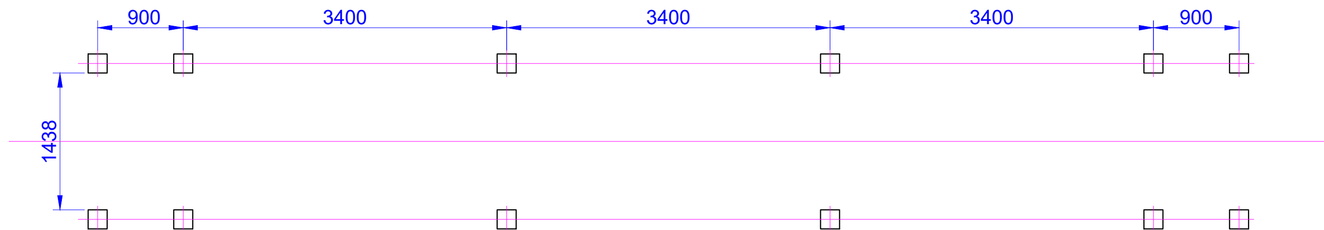
Схема фундаментов (свай)
